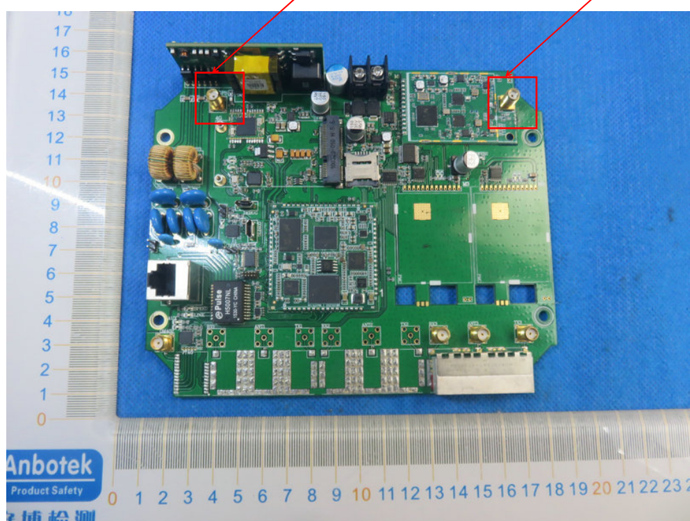
GPS Antenna
