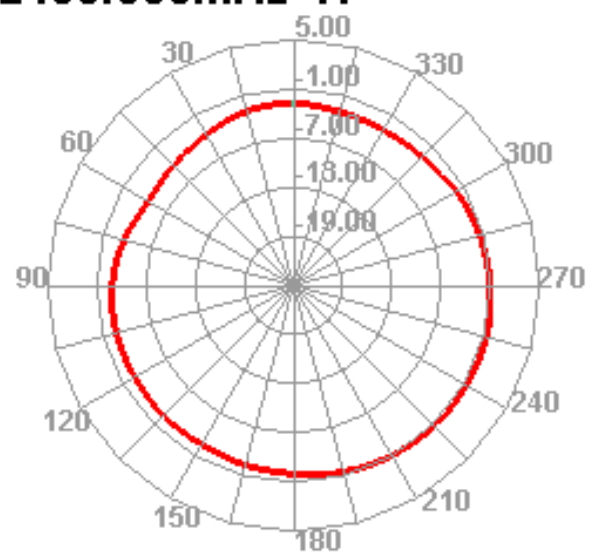
2450.000MHz H
