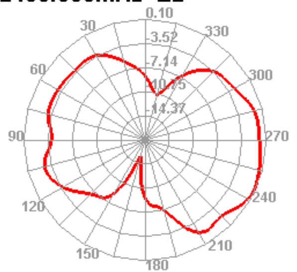
2450.000MHz E2
