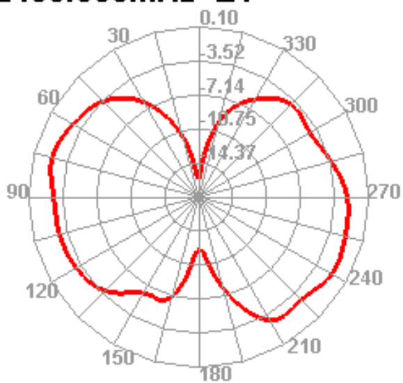
2450.000MHz E1
