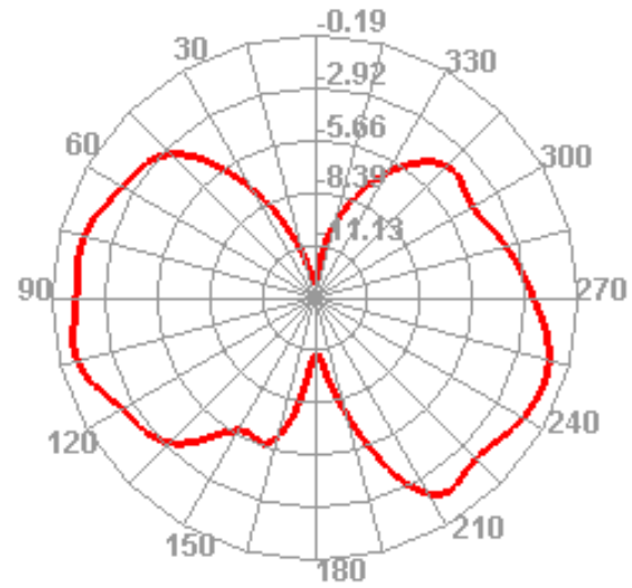
2500.000MHz E1
