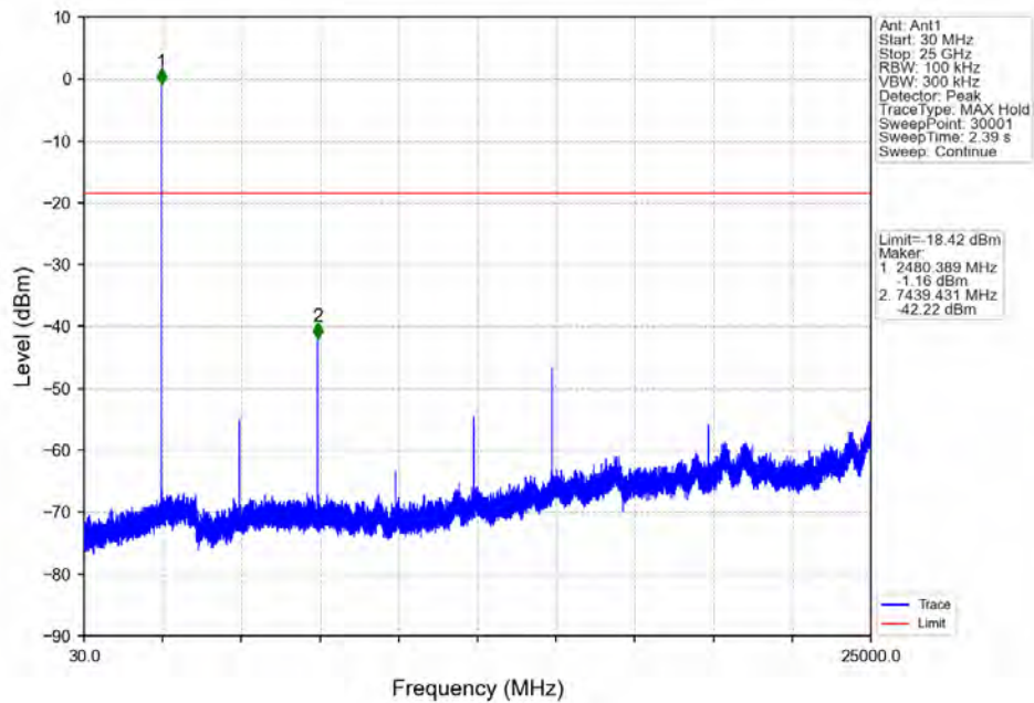
PI/4-QDPSK_HOPP_Ant1_NTNV
