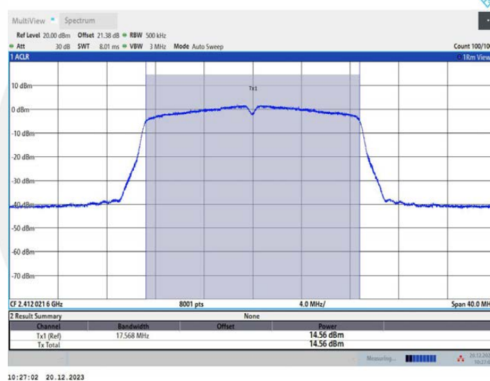
11N20MIMO_Ant3_2412
