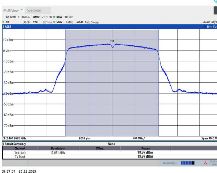
11G_Ant2_2462
