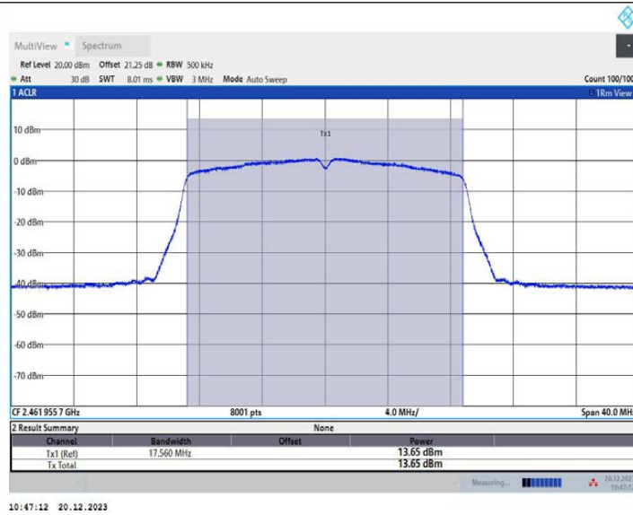
11N20MIMO_Ant3_2462
