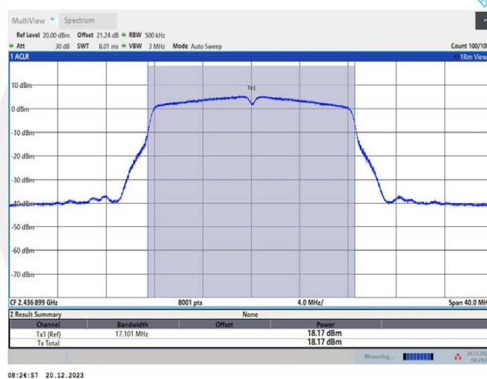
11G_Ant2_2437
