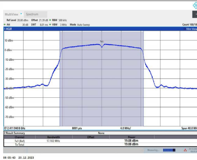
11G_Ant2_2412
