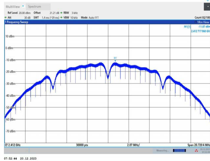
11B_Ant2_2412
