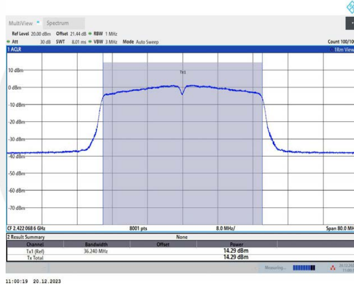
11N40MIMO_Ant3_2422
