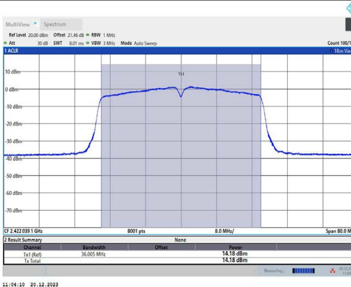
11N40MIMO_Ant4_2422
