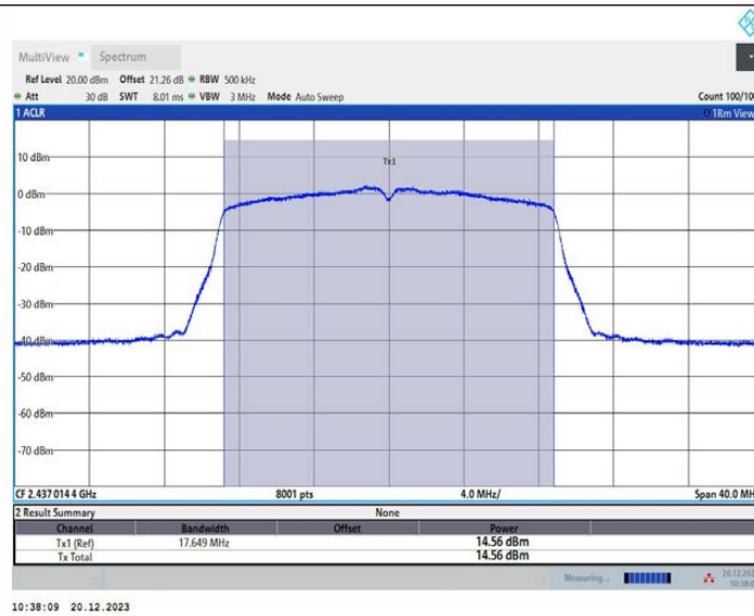
11N20MIMO_Ant4_2437
