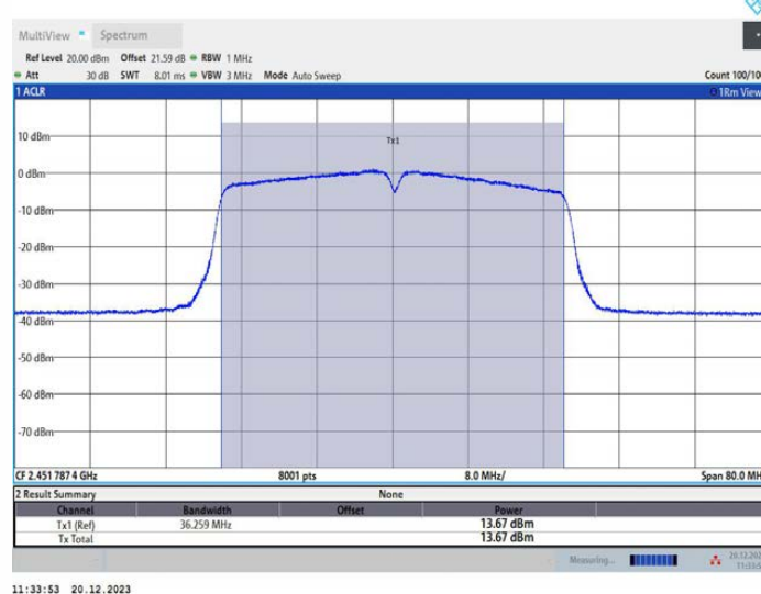
11N40MIMO_Ant4_2452
