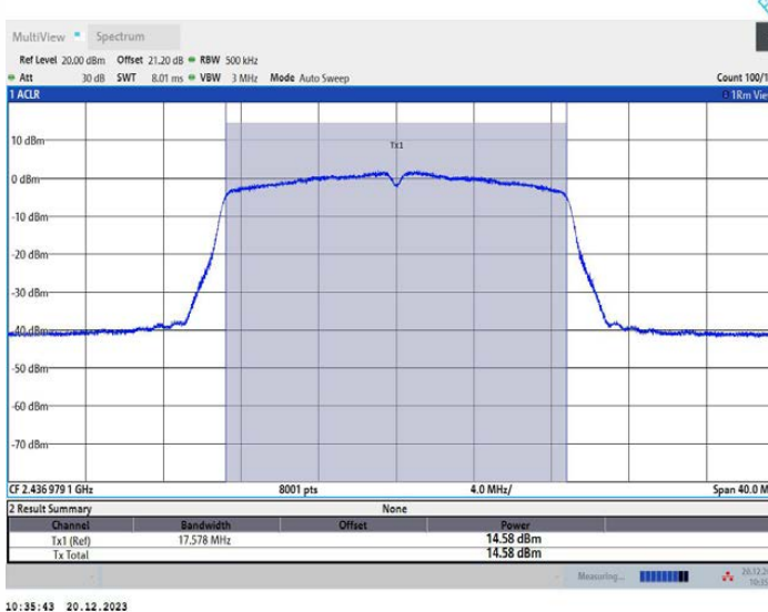
11N20MIMO_Ant3_2437
