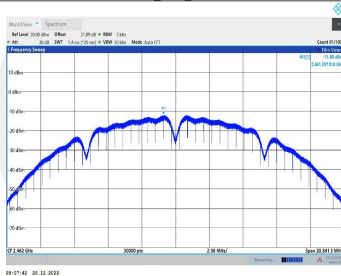
11B_Ant4_2462
