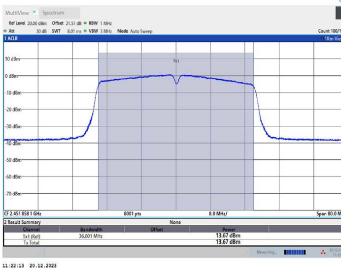
11N40MIMO_Ant2_2452
