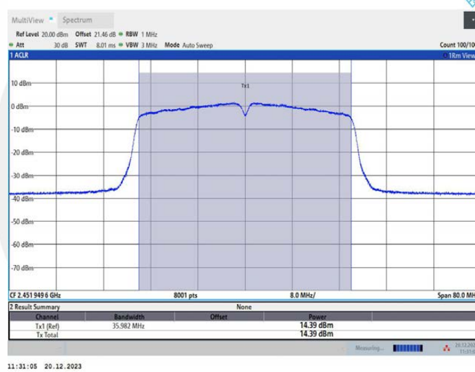
11N40MIMO_Ant4_2452
