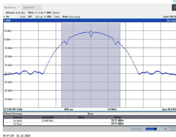
11B_Ant4_2462
