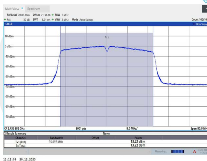
11N40MIMO_Ant2_2437
