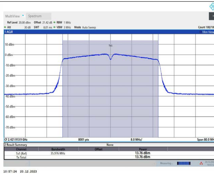
11N40MIMO_Ant2_2422
