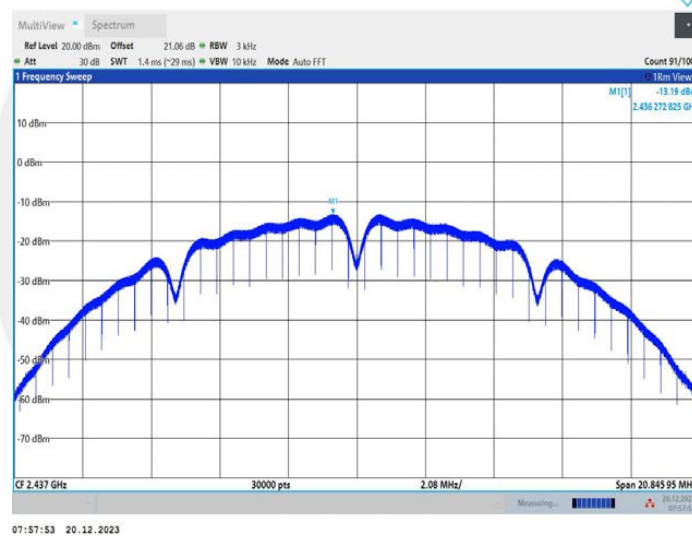
11B_Ant2_2437
