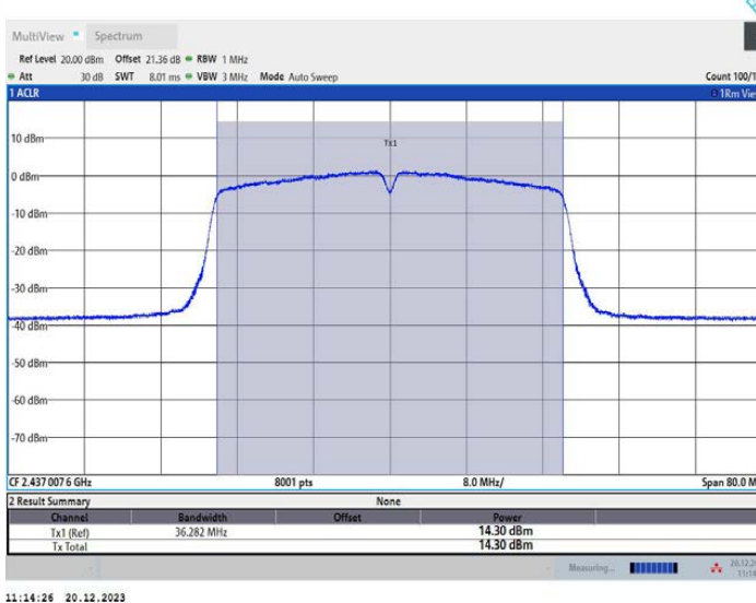
11N40MIMO_Ant3_2437
