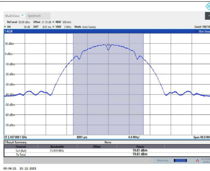
11B_Ant4_2437
