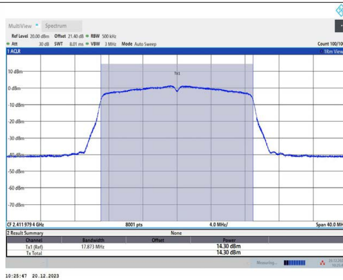
11N20MIMO_Ant2_2412
