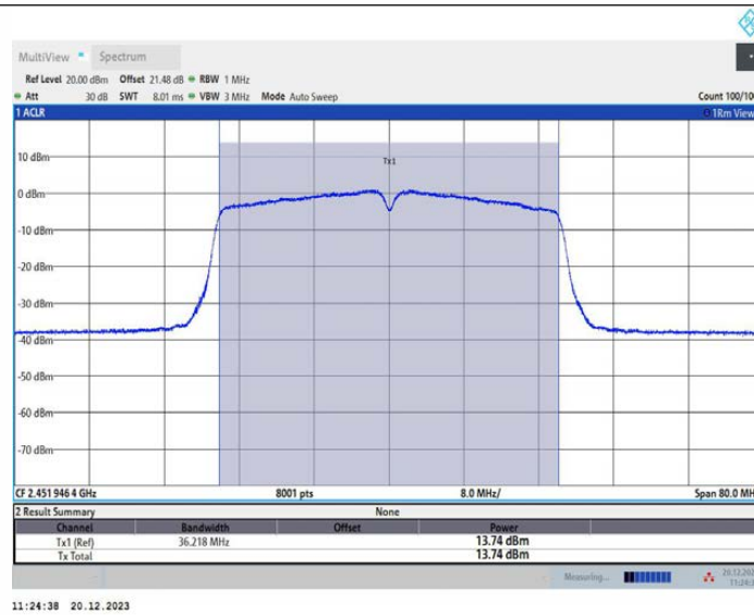
11N40MIMO_Ant3_2452
