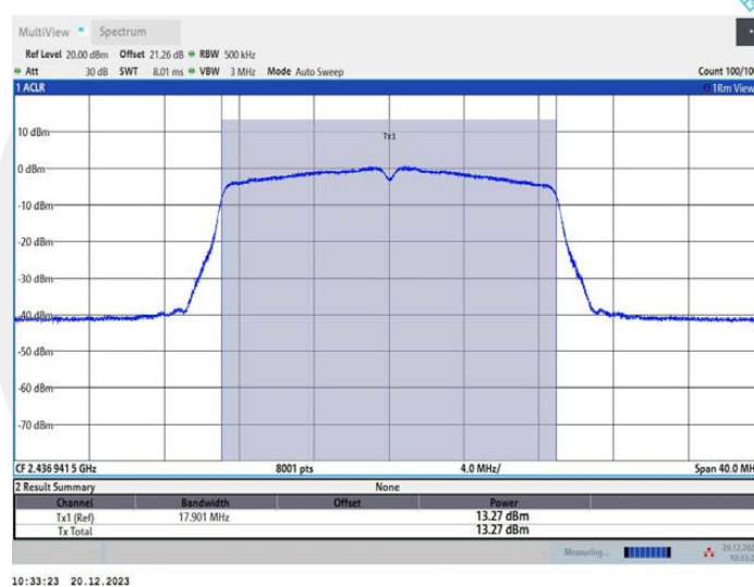
11N20MIMO_Ant2_2437
