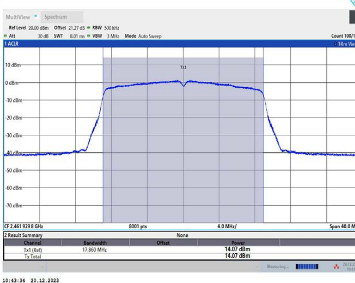
11N20MIMO_Ant2_2462
