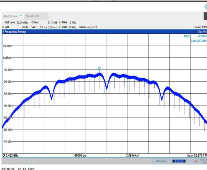
11B_Ant4_2462
