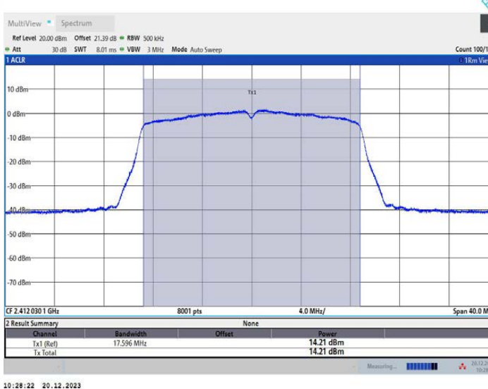
11N20MIMO_Ant4_2412
