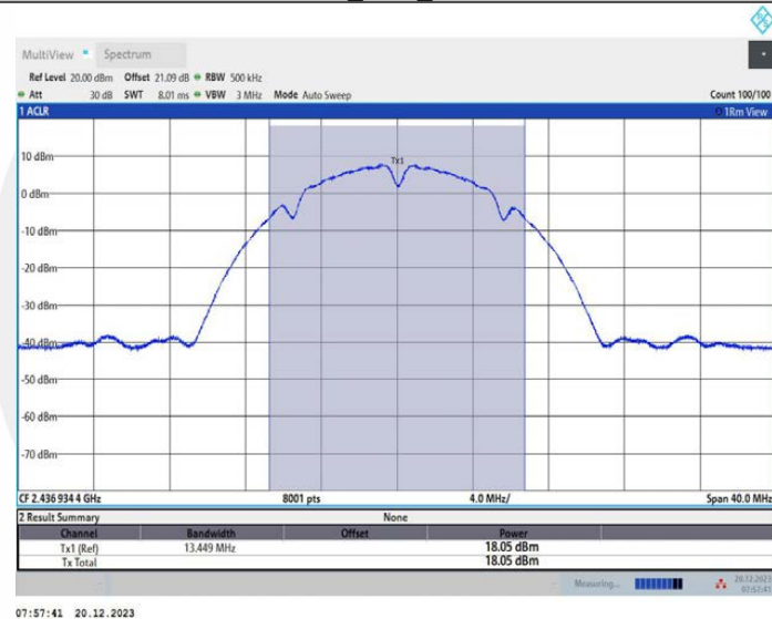
11B_Ant2_2437
