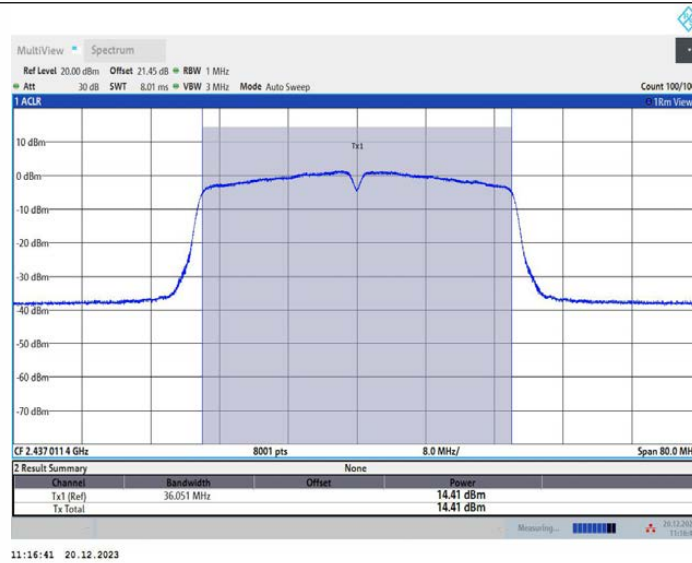
11N40MIMO_Ant4_2437
