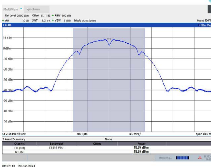
11B_Ant2_2462
