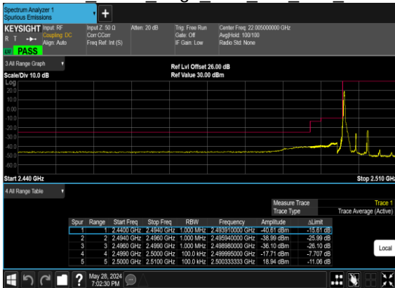
B2_N7(5M)_DFT-s- OFDM BPSK Edge 1RB Left Low CH
