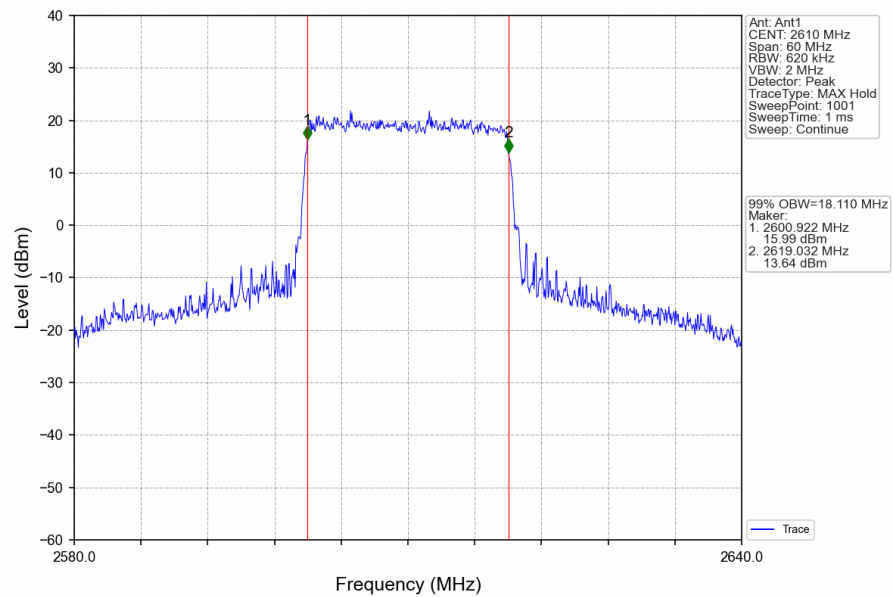
Band38_20MHz_16QAM_HCH_2610MHz_RB_100_0_NTNV
