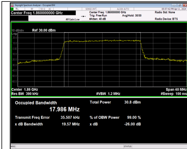
Band2-20MHz-16QAM-18700-100RB#0-PASS
