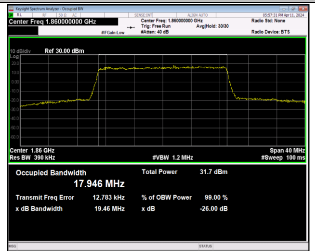
Band2-20MHz-QPSK-18700-100RB#0-PASS
