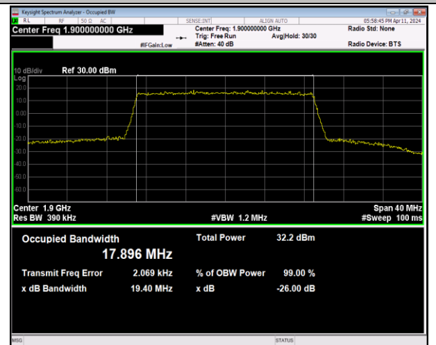
Band2-20MHz-QPSK-19100-100RB#0-PASS
