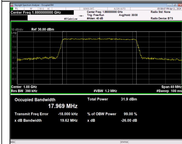
Band2-20MHz-QPSK-18900-100RB#0-PASS
