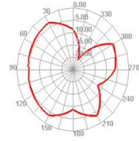
5810.000MHz H
