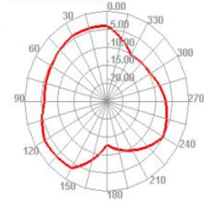
5270.000MHz E2
