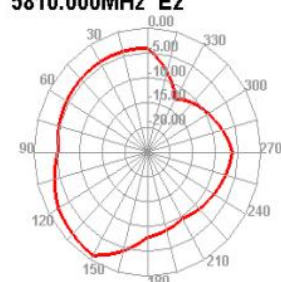
5810.000MHz E2
