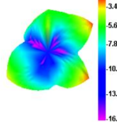
5270.000MHz E1
