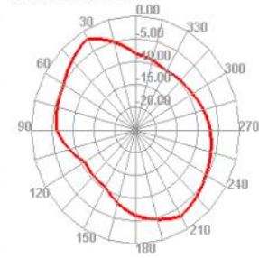
5270.000MHz H
