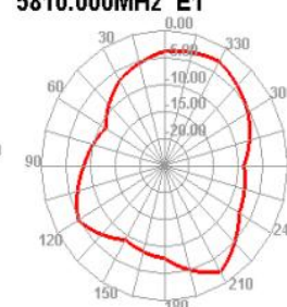
5810.000MHz E1
