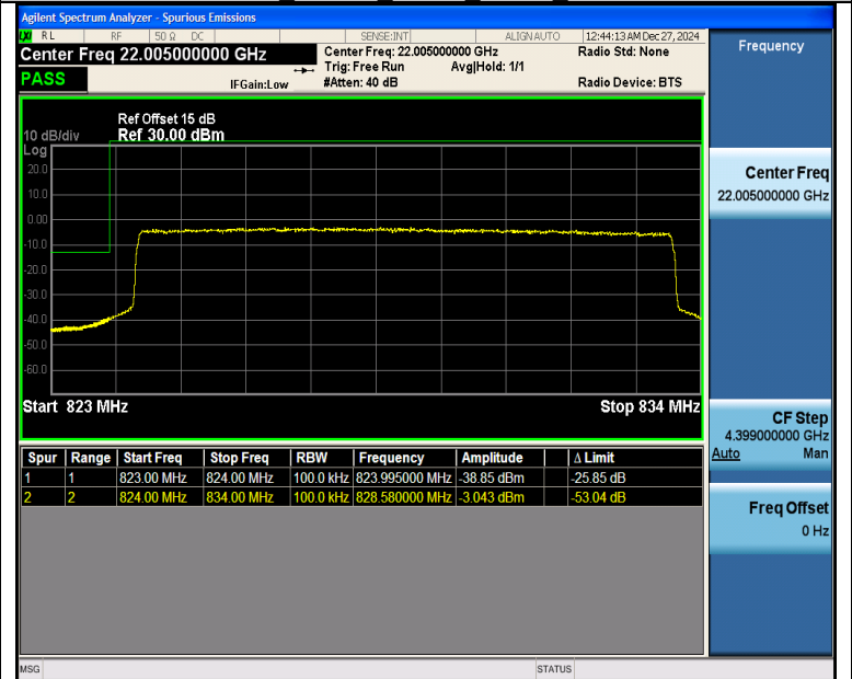
Band26 10MHz QPSK 26840 50RB#0
