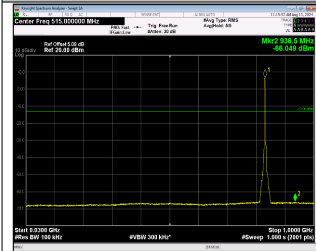
5-5-3MHz-5MHz-QPSK-QPSK-20501-20540-15RB#0-25 RB#0-30~1000MHz-PASS
