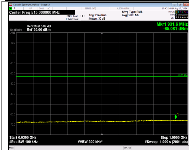
2-2-20MHz-20MHz-QPSK-QPSK-18902-19100-1RB#0-1 RB#99-30~1000MHz-PASS
