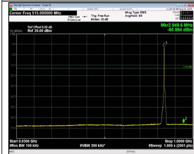
5-5-3MHz-5MHz-QPSK-QPSK-20586-20625-15RB#0-25 RB#0-30~1000MHz-PASS
