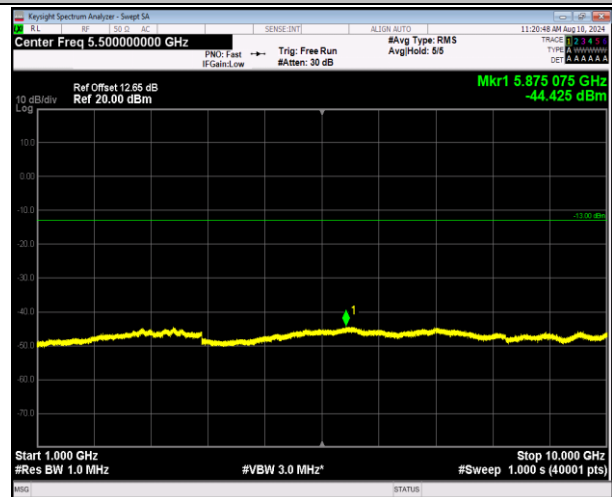
5-5-3MHz-5MHz-QPSK-QPSK-20586-20625-15RB#0-25RB #0-1000~10000MHz-PASS
