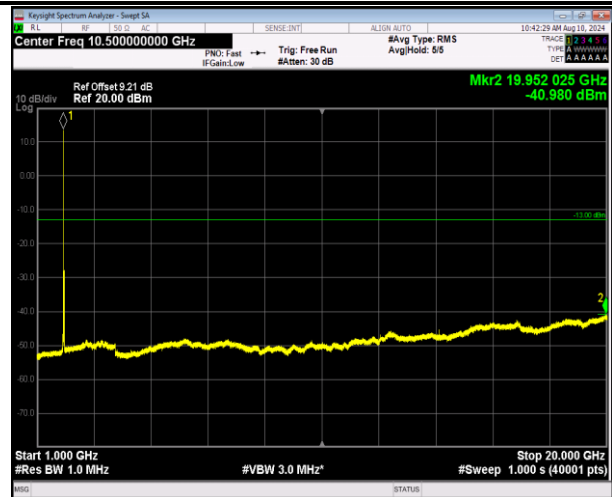
2-2-20MHz-20MHz-QPSK-QPSK-18902-19100-1RB#0-1RB #99-1000~20000MHz-PASS
