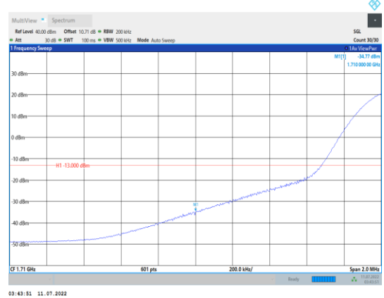
Band4-20MHz-QPSK-20050-1RB#0
