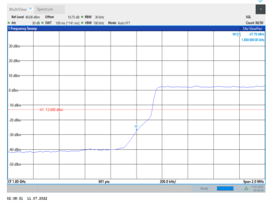
Band2-3MHz-QPSK-18615-15RB#0
