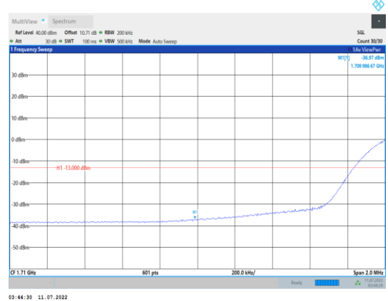
Band4-20MHz-QPSK-20050-100RB#0
