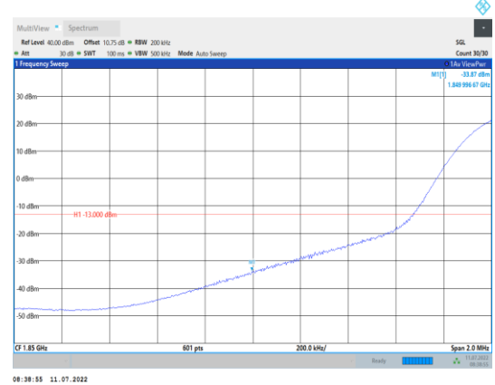
Band2-20MHz-QPSK-18700-1RB#0
