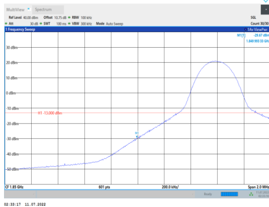
Band2-10MHz-QPSK-18650-1RB#0
