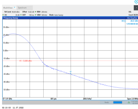
Band2-15MHz-16QAM-19125-1RB#74
