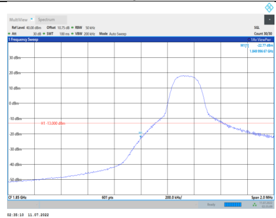
Band2-5MHz-QPSK-18625-1RB#0
