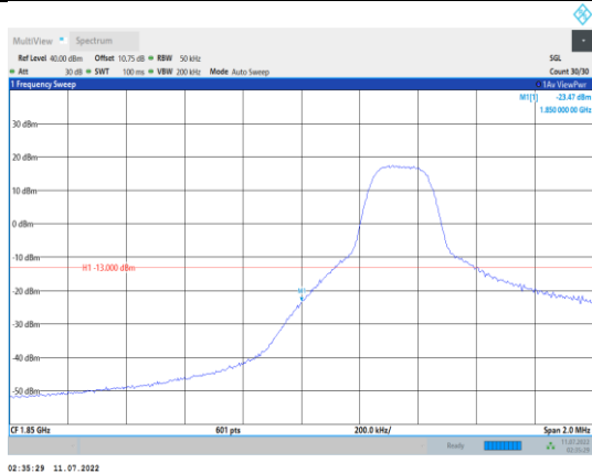
Band2-5MHz-16QAM-18625-1RB#0
