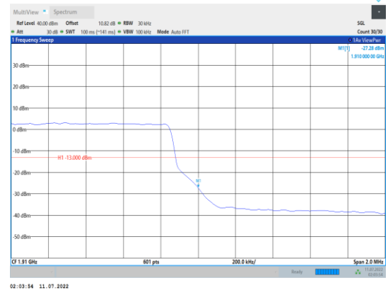
Band2-3MHz-QPSK-19185-15RB#0
