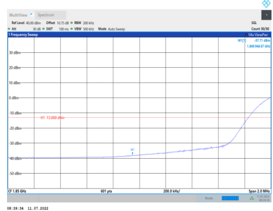
Band2-20MHz-QPSK-18700-100RB#0
