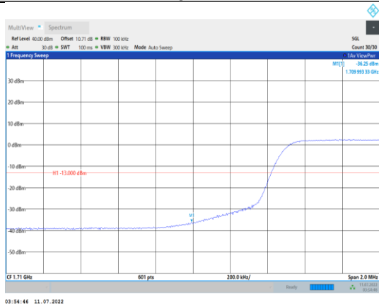
Band4-10MHz-QPSK-20000-50RB#0
