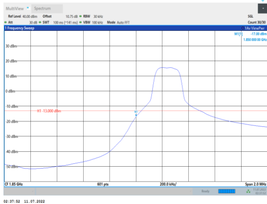
Band2-3MHz-QPSK-18615-1RB#0
