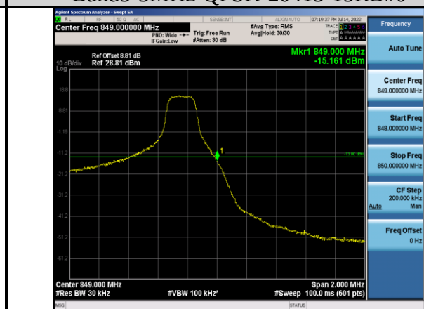
Band5-3MHz-QPSK-20635-1RB#14
