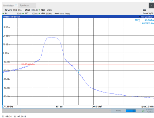
Band2-5MHz-QPSK-19175-1RB#24
