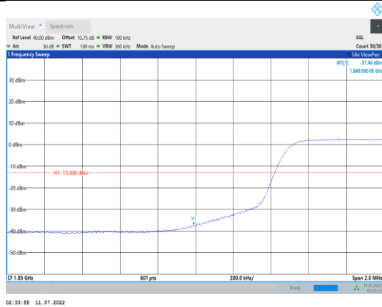
Band2-10MHz-QPSK-18650-50RB#0
