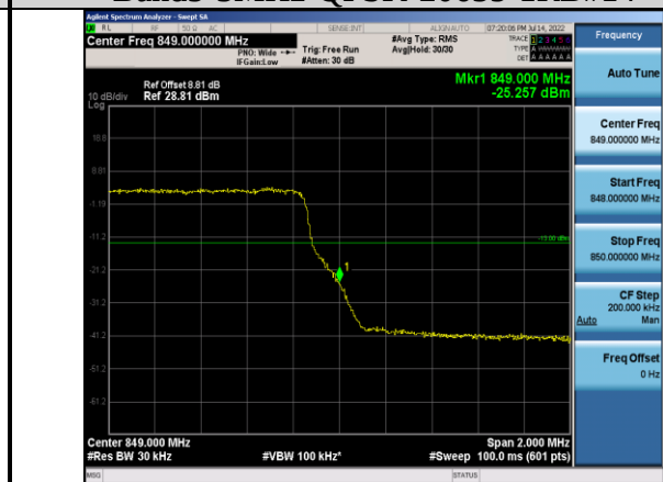
Band5-3MHz-QPSK-20635-15RB#0
