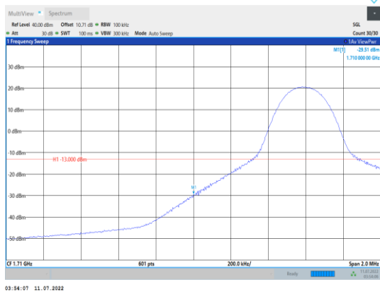
Band4-10MHz-QPSK-20000-1RB#0
