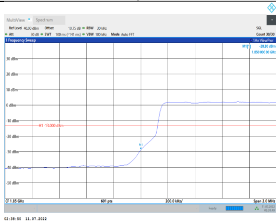
Band2-3MHz-16QAM-18615-15RB#0
