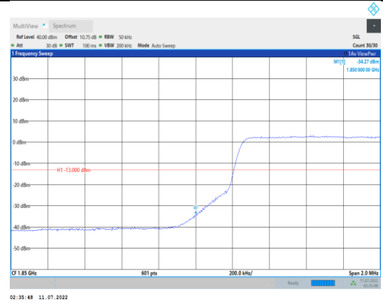
Band2-5MHz-QPSK-18625-25RB#0
