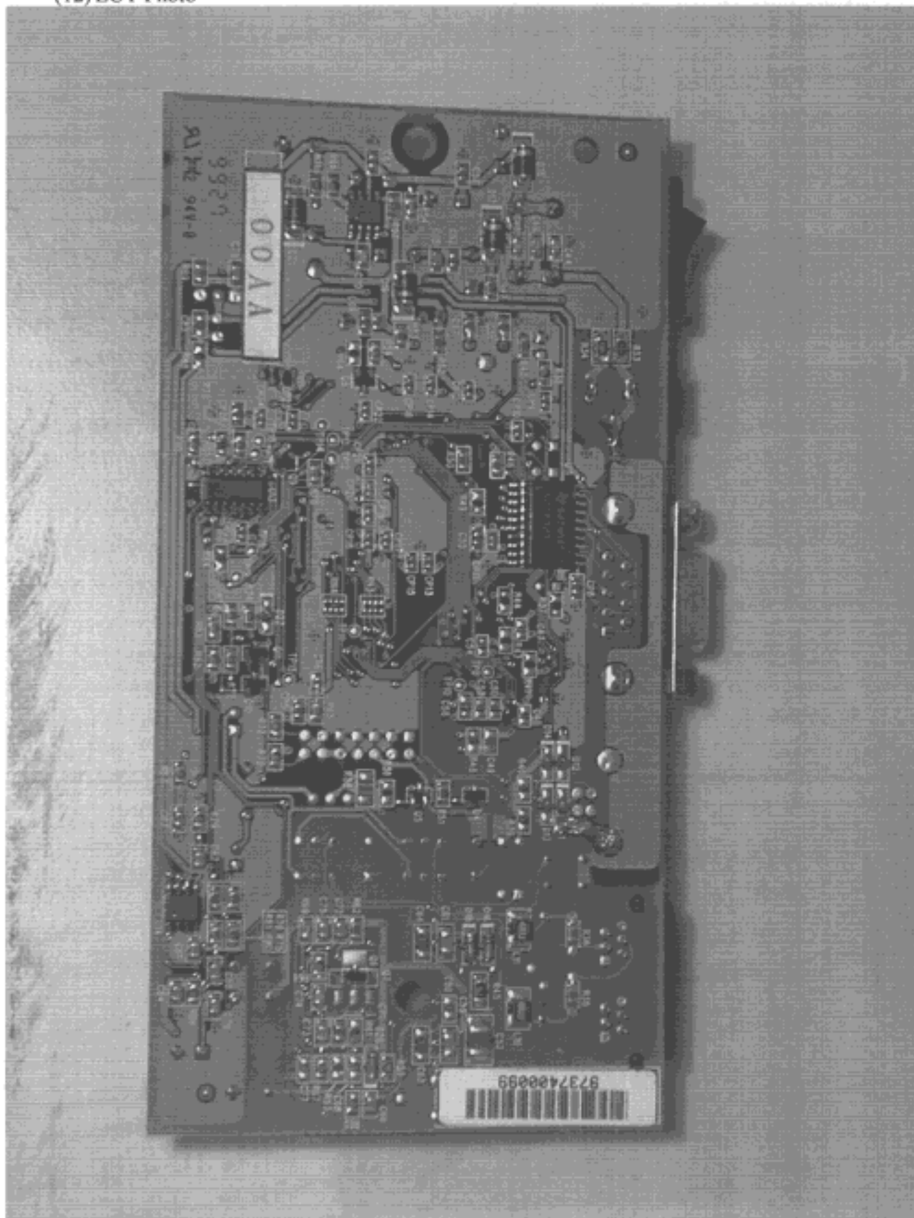
(12) EUT Photo
