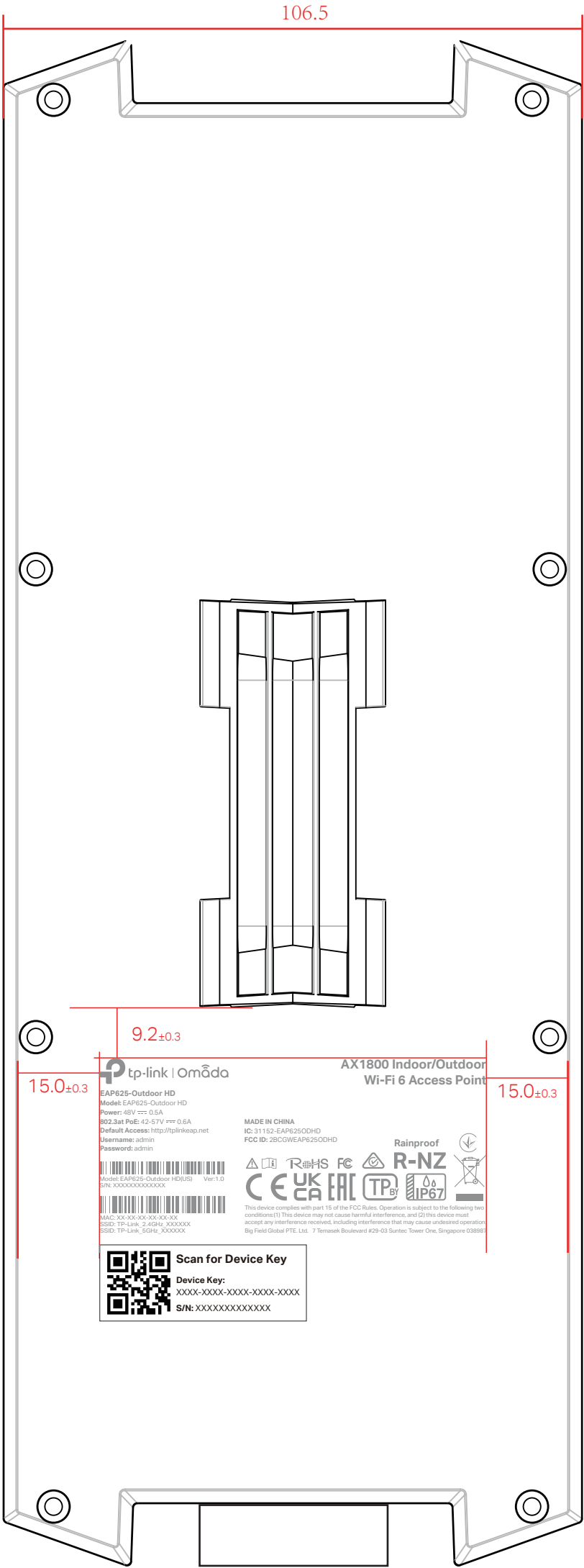
尺寸图
