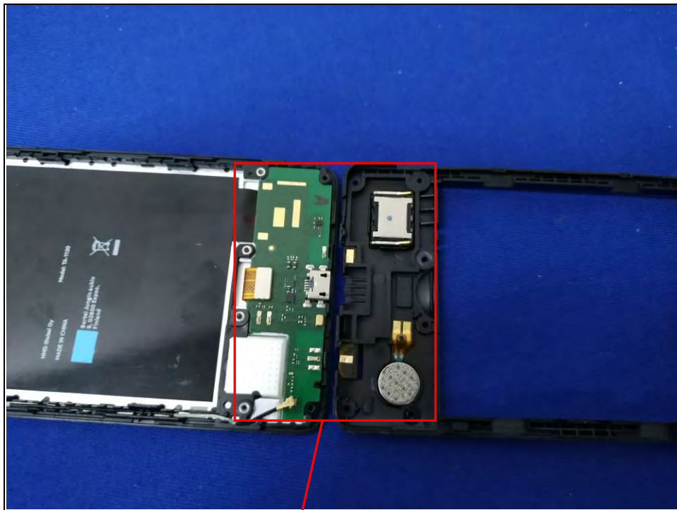
WWAN Antenna
