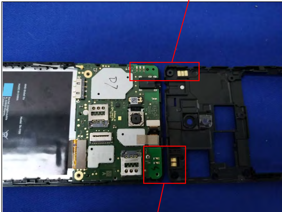
BT/WIFI Antenna
