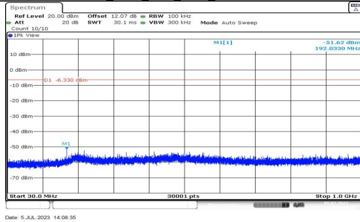
BLE 125K Ant3 2440 30-1000
