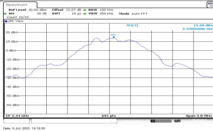
BLE 500K Ant3 2440 0-Reference
