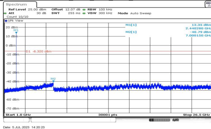
BLE 500K Ant3 2440 1000-26500
