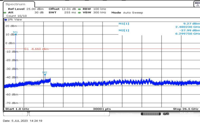
BLE_500K_Ant3_2480_1000-26500
