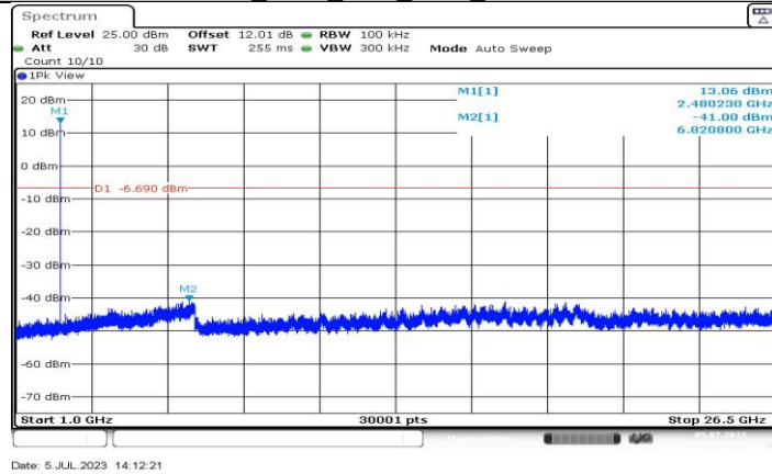
BLE 125K Ant3 2480 1000-26500
