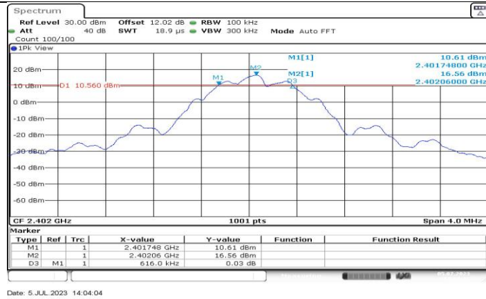
BLE 125K Ant3 2402
