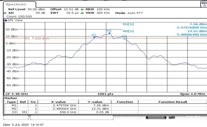
BLE 125K Ant3 2480
