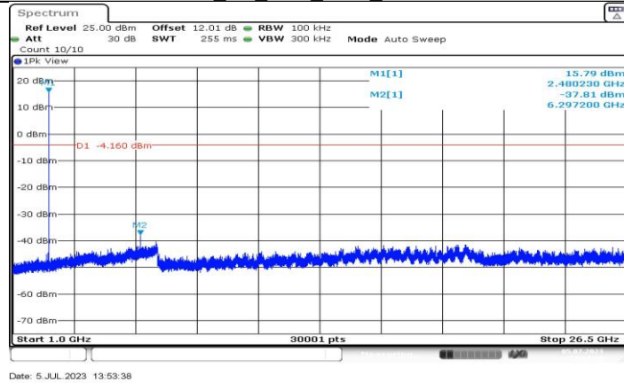
BLE 1M Ant3 2480 1000-26500
