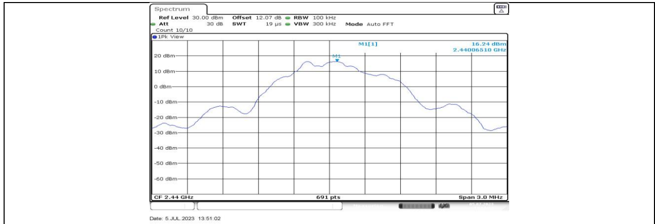
BLE 1M Ant3 2440 0-Reference
