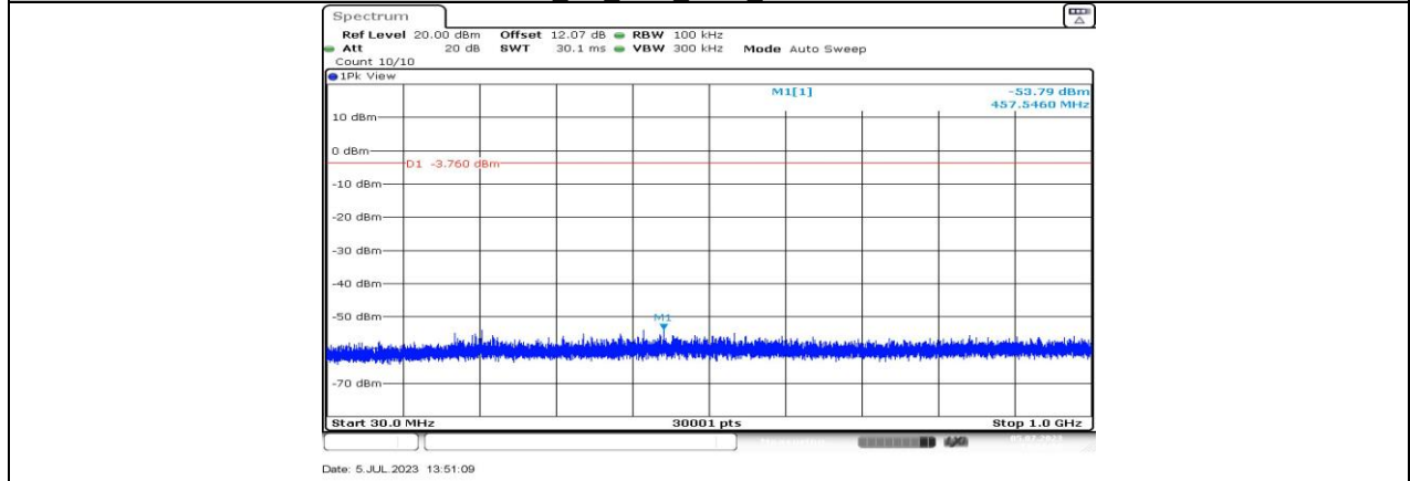
BLE 1M Ant3 2440 30-1000
