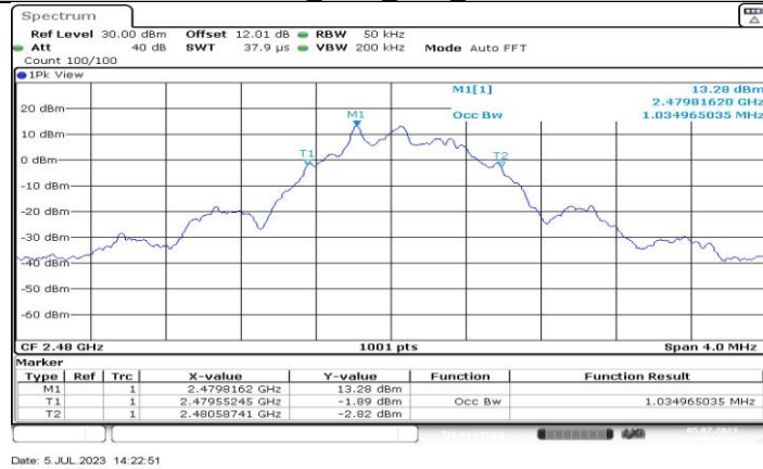
BLE_500K_Ant3_2480
