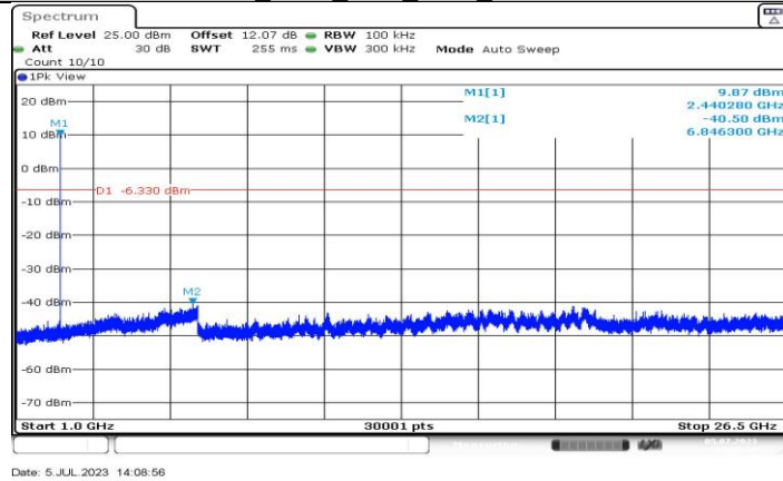
BLE 125K Ant3 2440 1000-26500
