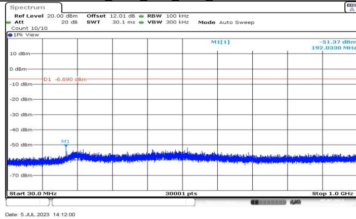
BLE 125K Ant3 2480 30-1000
