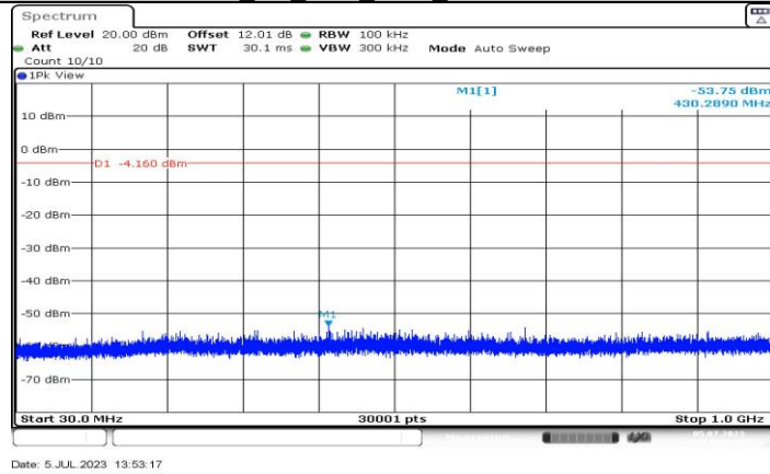
BLE 1M Ant3 2480 30-1000
