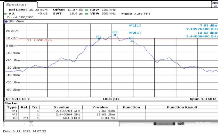
BLE 125K Ant3 2440
