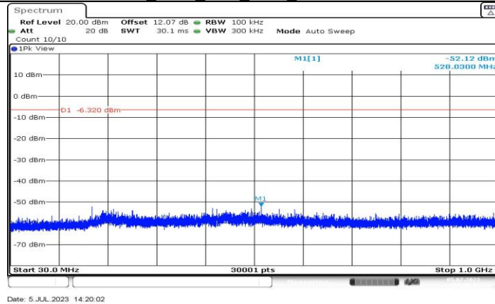
BLE 500K Ant3 2440 30-1000
