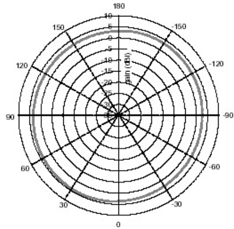
R380.900.903 H-PLANE
