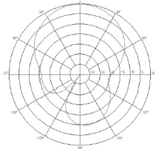
R380.900.909, 2.4 GHz, E-PLANE
