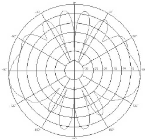
R380.900.908, 4.9 GHz, E-PLANE
