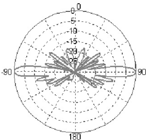
R380.600.200 E-PLANE
