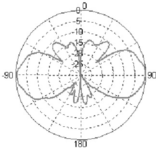
R380.700.206 E-PLANE
