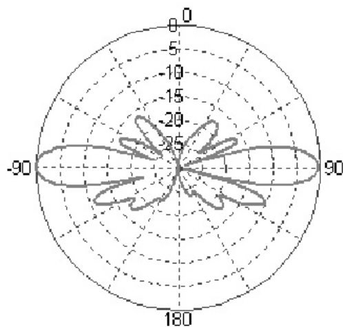
R380.500.220 E-PLANE
