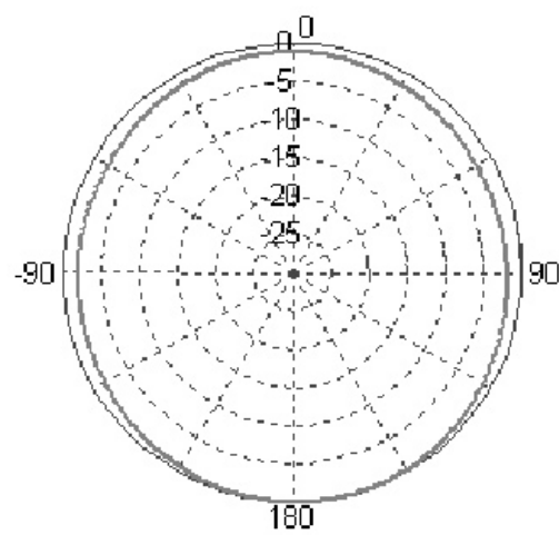
R380.600.200 H-PLANE
