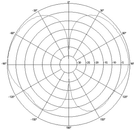
R380.500.501 E-PLANE
