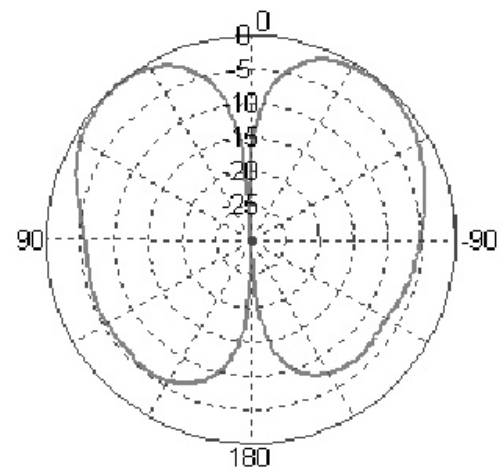
R380.900.500, 5 GHz, E-PLANE
