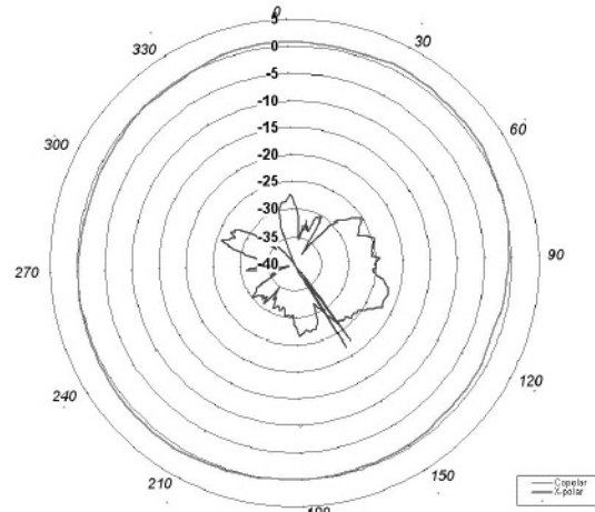
LPT2400NMOHF H-PLANE
