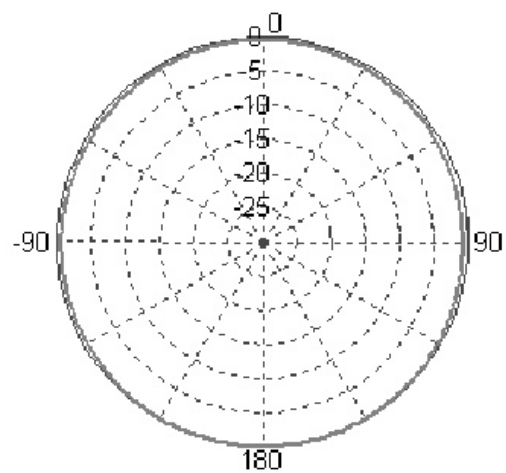
R380.500.219 H-PLANE
