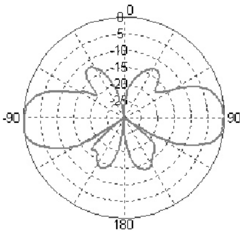
R380.500.219 E-PLANE
