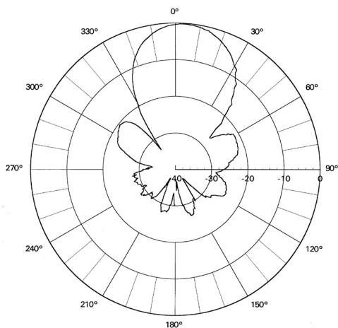
PA4142400 E-PLANE
