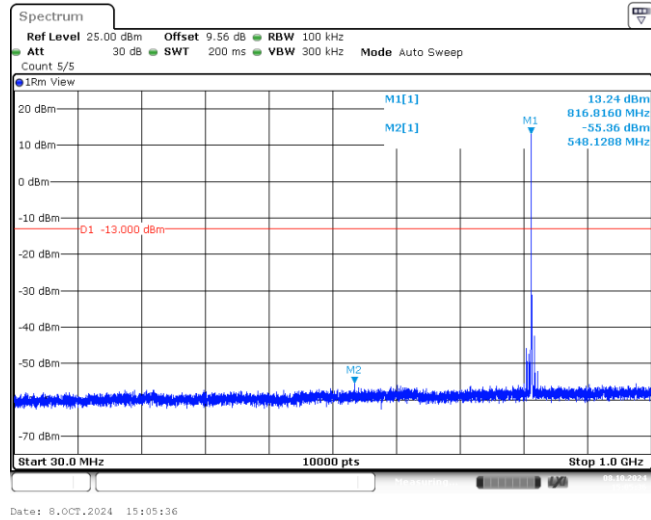
Band26-5MHz-QPSK-26740-1-0-Low-30-1000--55.36-PASS
