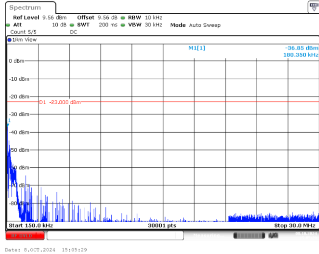
Band26-5MHz-QPSK-26740-1-0-Low-0.15-30--36.85-PASS
