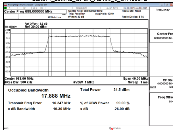
Band71_20MHz_QPSK_RB100_0_CH133372
