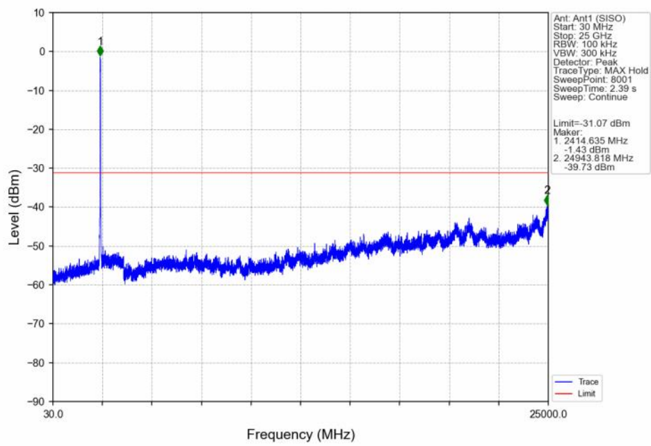
802.11n(HT40)_MCH_2437MHz_Ant1 (SISO)_NTNV
