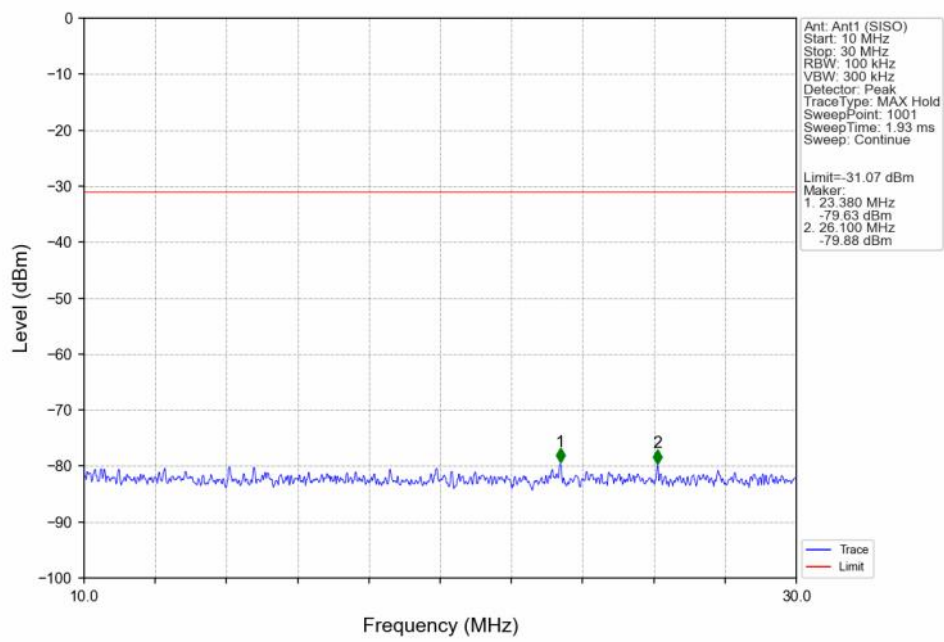
802.11n(HT40)_HCH_2452MHz_Ant1 (SISO)_NTNV
