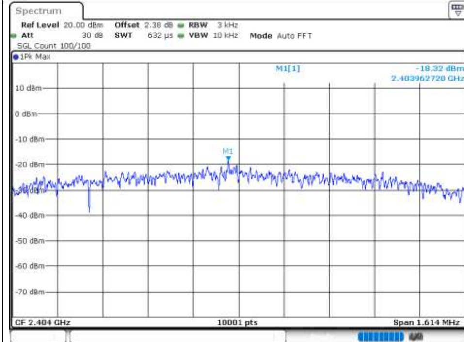
Test Graphs PSD NVNT BLE 2M 2404MHz Ant1
