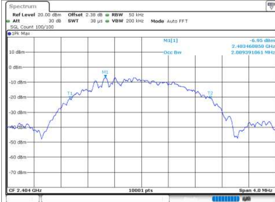
Test Graphs OBW NVNT BLE 2M 2404MHz Ant1
