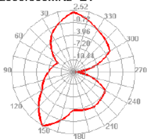
2500.000MHz E1
