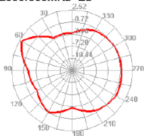
2500.000MHz E2
