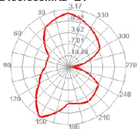
2450.000MHz E1
