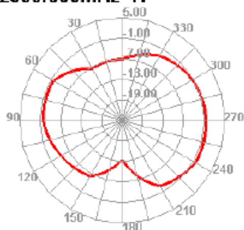
2500.000MHz H
