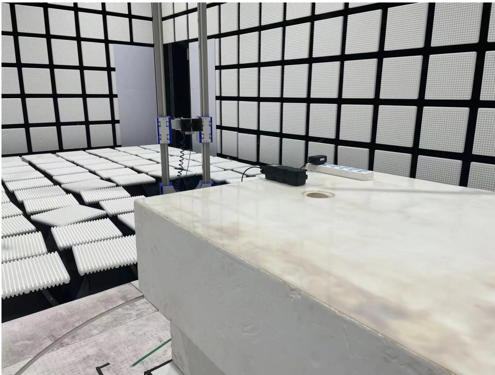
RE 1GHz-18GHz
