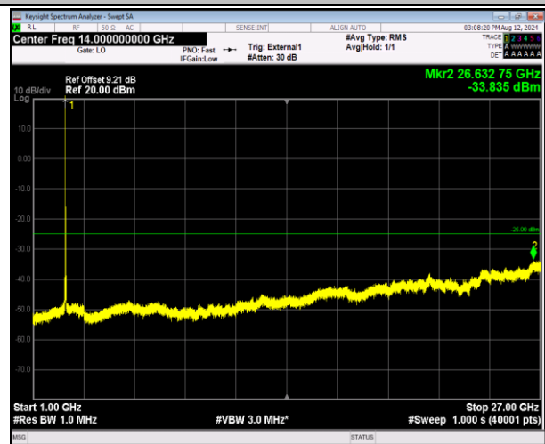
41-41-20MHz-10MHz-QPSK-QPSK-41391-41535-1RB#0-0 RB#0-1000~27000MHz-PASS
