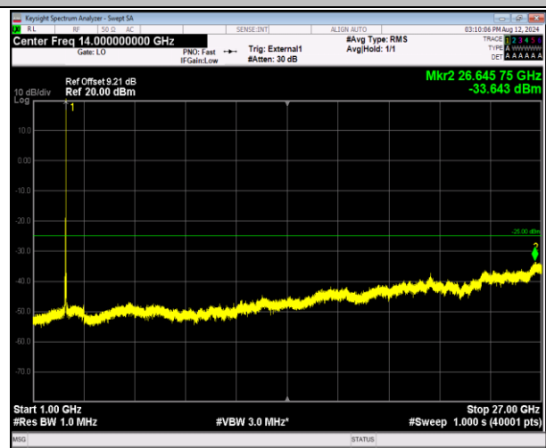
41-41-20MHz-10MHz-QPSK-QPSK-41391-41535-1RB#99- 0RB#0-1000~27000MHz-PASS
