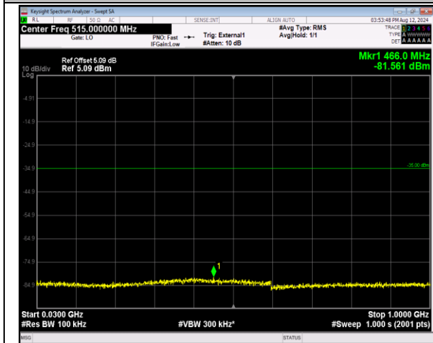
41-41-20MHz-20MHz-QPSK-QPSK-40521-40719-1RB#0 -0RB#0-30~1000MHz-PASS
