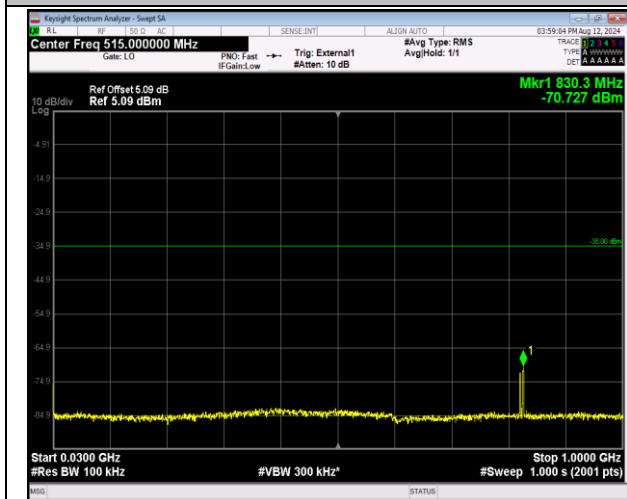
41-41-20MHz-20MHz-QPSK-QPSK-40521-40719-100RB #0-100RB#0-30~1000MHz-PASS
