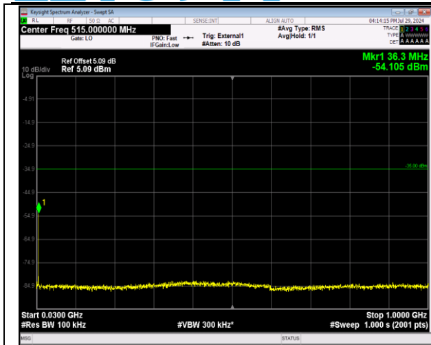
41-41-20MHz-10MHz-64QAM-64QAM-40571-40715-1RB #99-0RB#0-30~1000MHz-PASS
