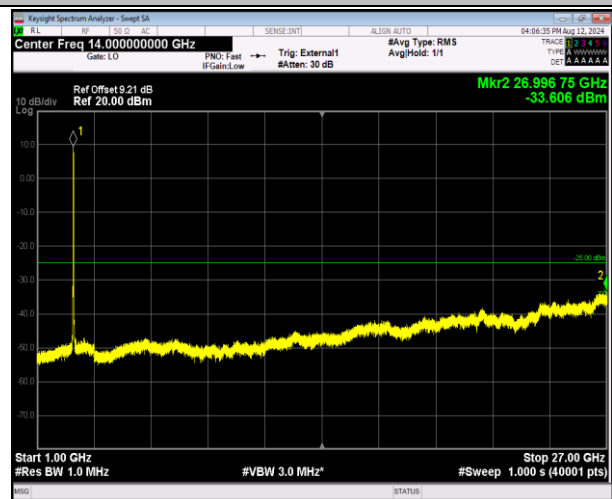
41-41-20MHz-20MHz-QPSK-QPSK-41292-41490-100RB#0 -100RB#0-1000~27000MHz-PASS
