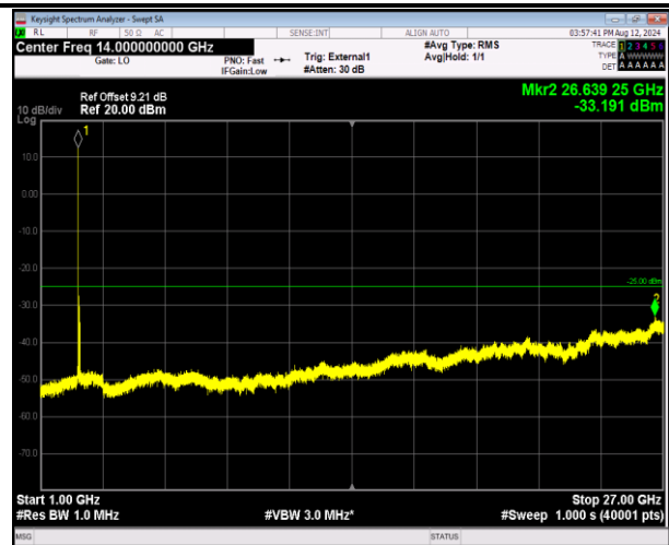
41-41-20MHz-20MHz-QPSK-QPSK-40521-40719-1RB#0-1 RB#99-1000~27000MHz-PASS
