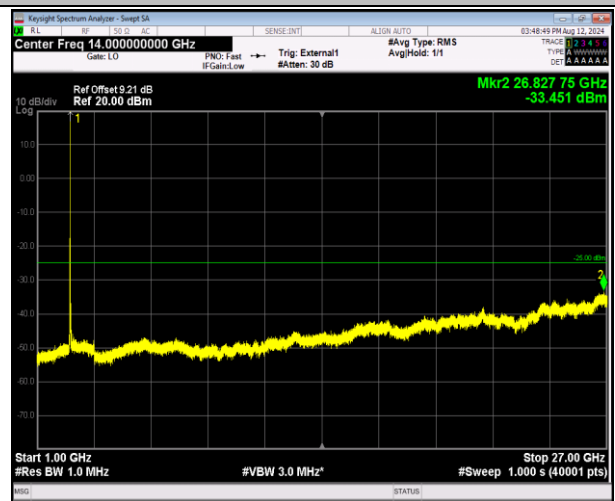
41-41-20MHz-20MHz-QPSK-QPSK-39750-39948-1RB#99- 0RB#0-1000~27000MHz-PASS
