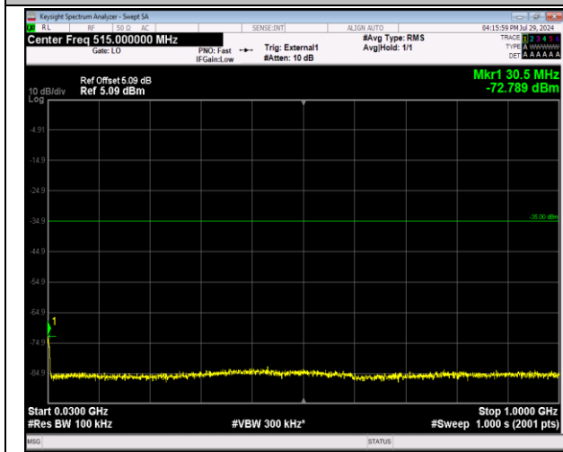
41-41-20MHz-10MHz-64QAM-64QAM-40571-40715-100 RB#0-50RB#0-30~1000MHz-PASS
