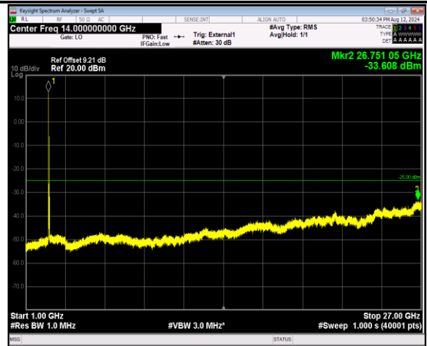
41-41-20MHz-20MHz-QPSK-QPSK-39750-39948-1RB#0-1 RB#99-1000~27000MHz-PASS
