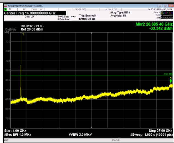
41-41-20MHz-20MHz-QPSK-QPSK-41292-41490-1RB#99- 0RB#0-1000~27000MHz-PASS
