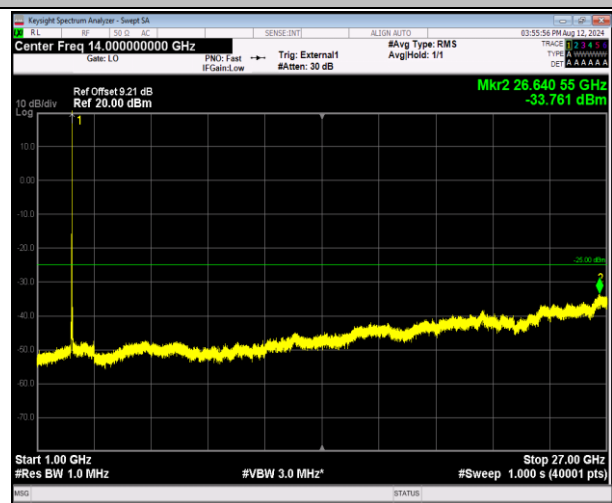
41-41-20MHz-20MHz-QPSK-QPSK-40521-40719-1RB#99- 0RB#0-1000~27000MHz-PASS
