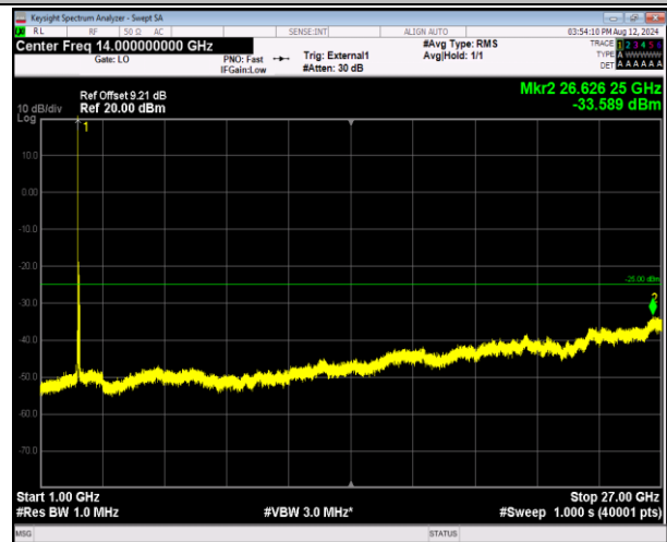
41-41-20MHz-20MHz-QPSK-QPSK-40521-40719-1RB#0-0 RB#0-1000~27000MHz-PASS
