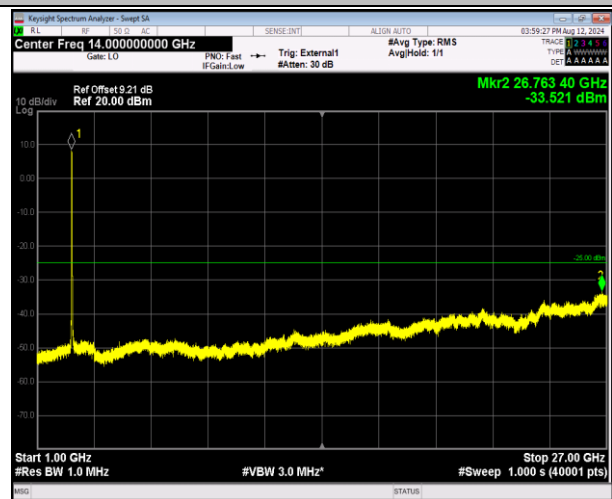
41-41-20MHz-20MHz-QPSK-QPSK-40521-40719-100RB#0 -100RB#0-1000~27000MHz-PASS
