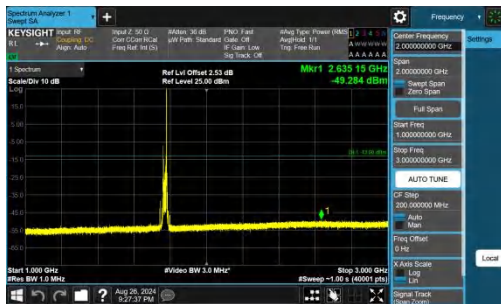
Band66-20MHz-QPSK-132572-1RB#99-1000~3000-PASS
