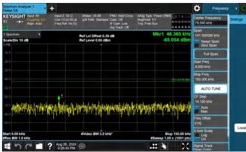
Band66-20MHz-QPSK-132572-1RB#0-0.009~0.15-PASS
