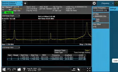
Band66-20MHz-QPSK-132072-1RB#99-PASS
