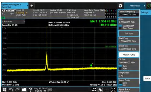
Band66-20MHz-QPSK-132072-1RB#99-1000~3000-PASS
