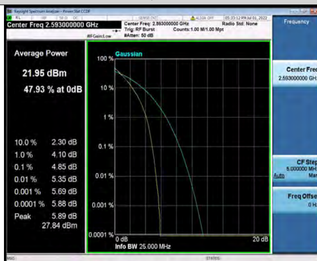
Band41-20MHz-QPSK-41490-1RB#0
