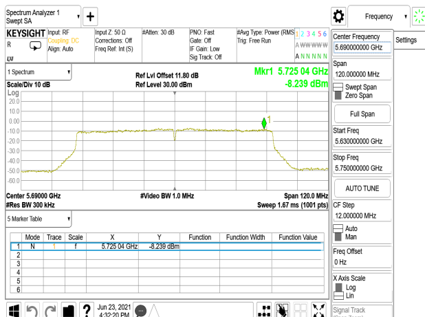
802.11ac_80MHz_Chain1_5690MHz_UNII 3
