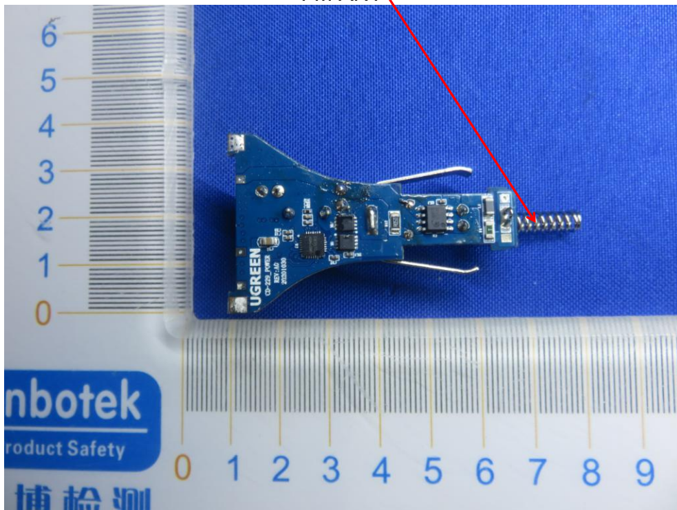
FM ANT
