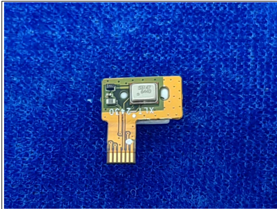
EUT-15
