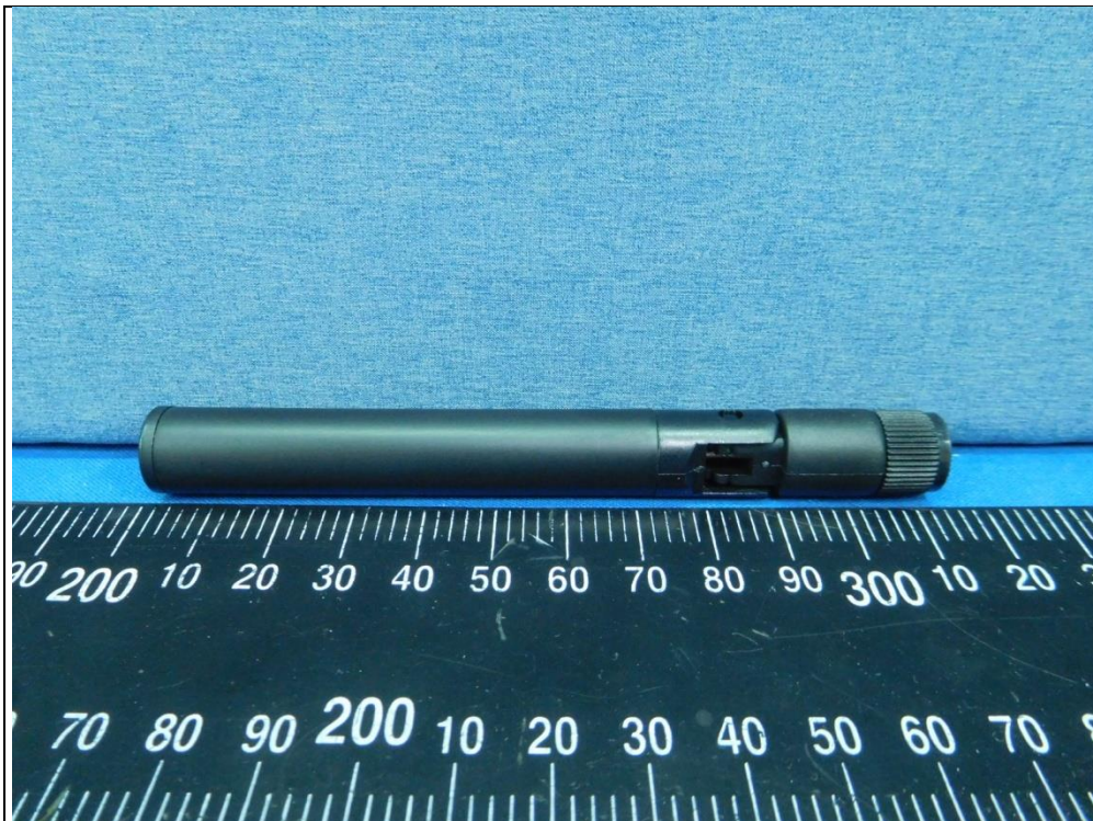
Dipole Antenna (Brand: LSR / Model: 001-0012)
