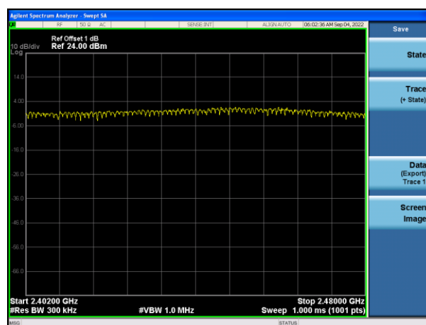
Mode 3
