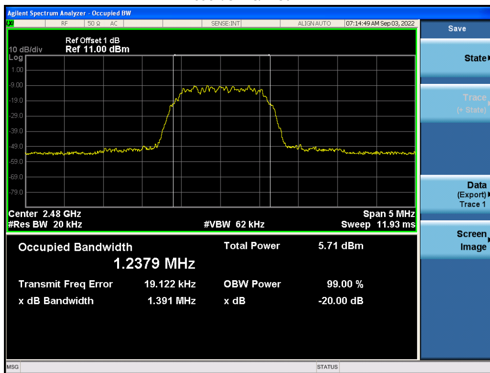
Mode2/CH78/2480MHz
