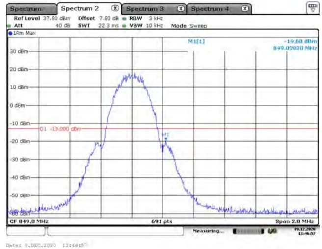
EGPRS 850, Right Band Edge
