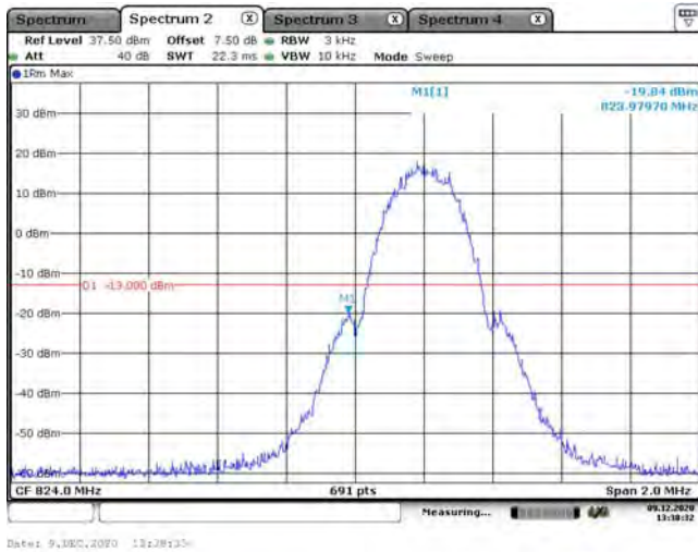
EGPRS 850, Left Band Edge
