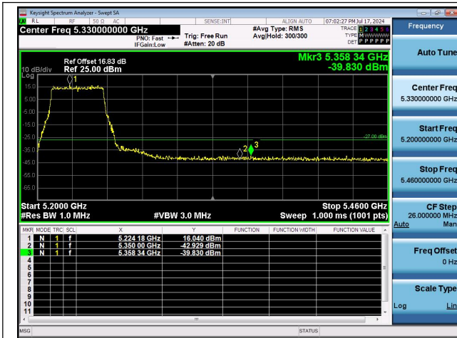
11AX40MIMO-Ant0-5230-PASS
