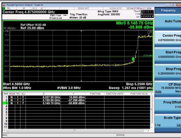
11AX80MIMO-Ant0-5210-PASS
