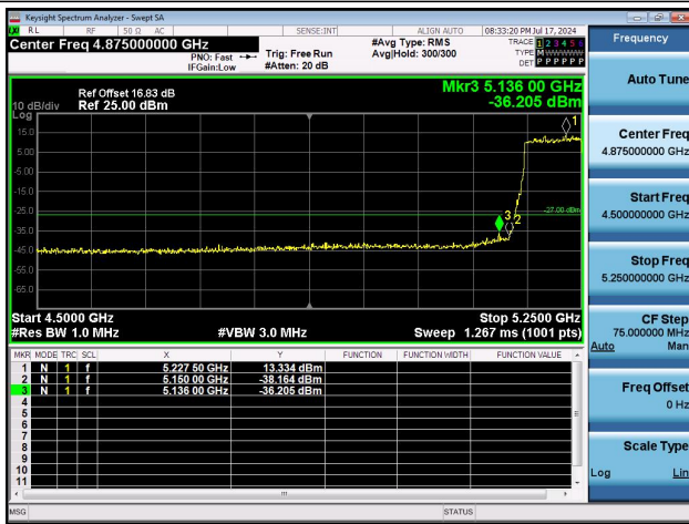
11AX80MIMO-Ant1-5210-PASS
