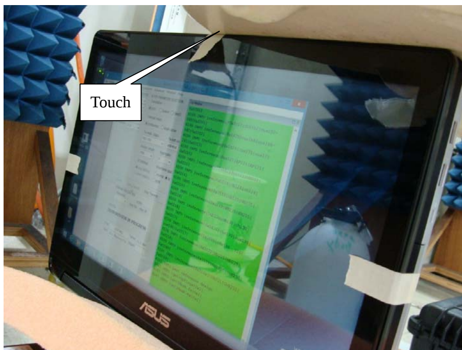
EUT Top
