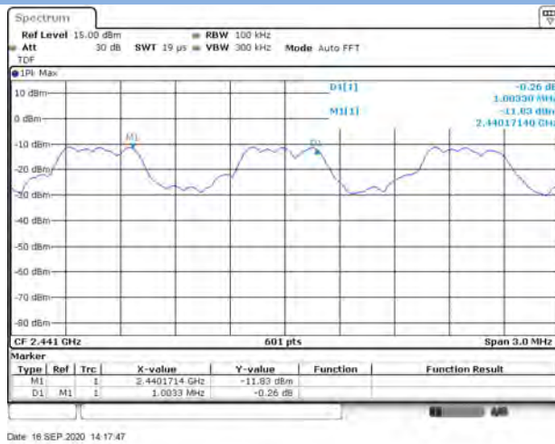
GFSK
