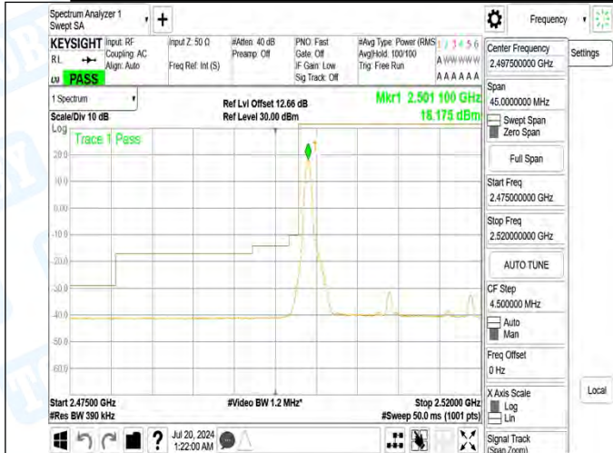
Band7_20MHz_16QAM_20850_100RB#0
