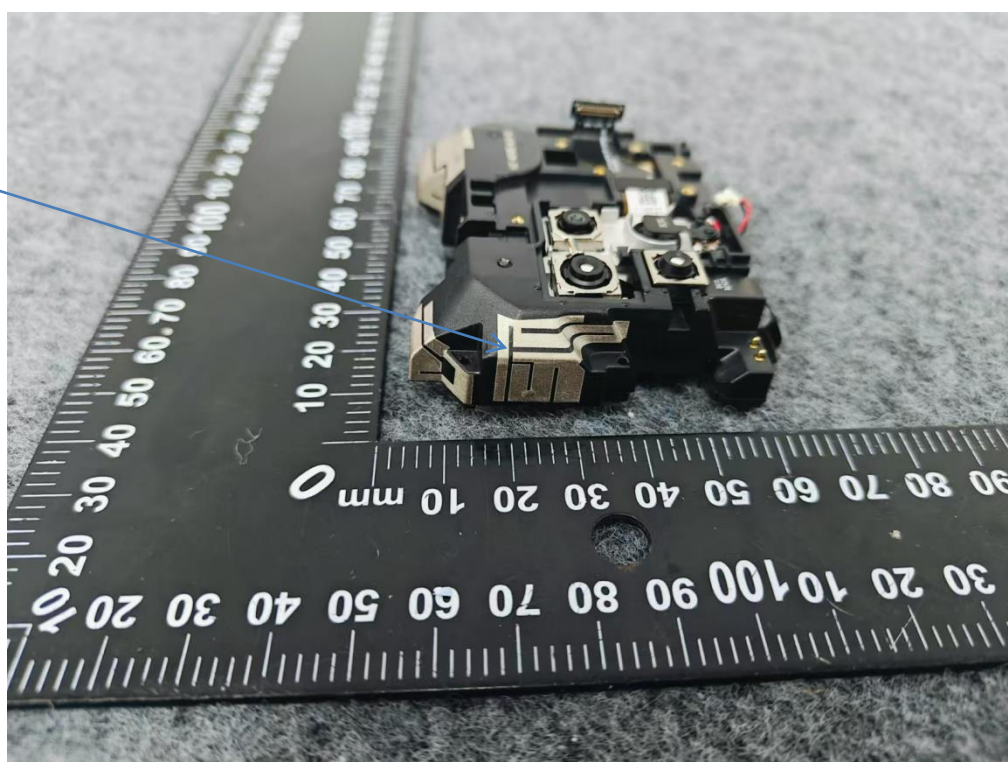
GPS/WIFI/BT ANT
