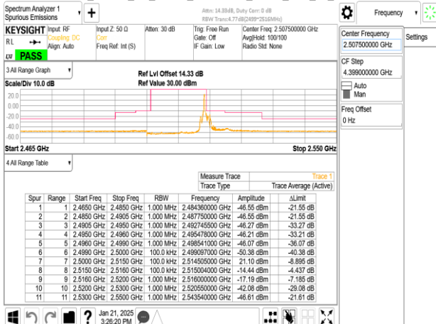
Band7_15MHz_CP_OFDM_SCS15kHz_QPSK_RB1_78_CH501500
