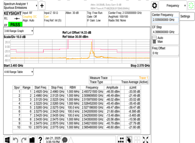
Band7_15MHz_CP_OFDM_SCS15kHz_QPSK_RB1_78_CH507000
