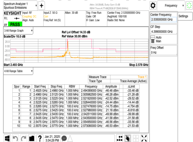
Band7_15MHz_CP_OFDM_SCS15kHz_QPSK_RB1_78_CH507000
