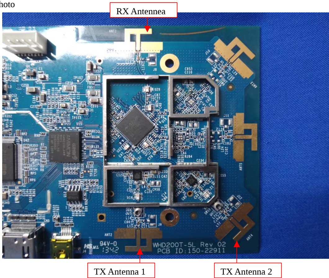
(10) EUT Photo
