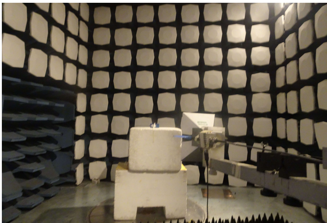
1GHz-18GHz
