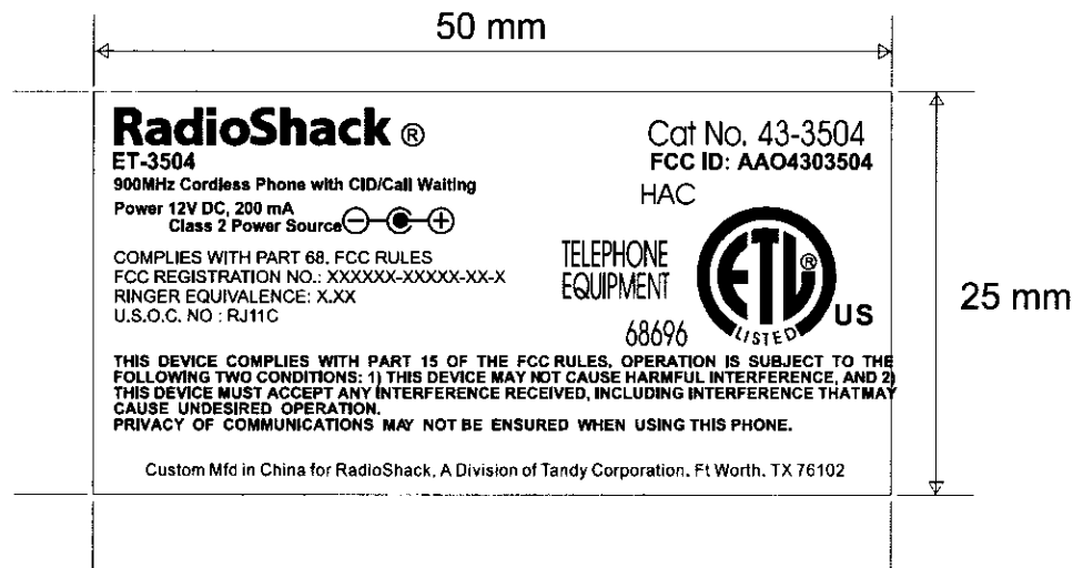
SCALE 2:1
