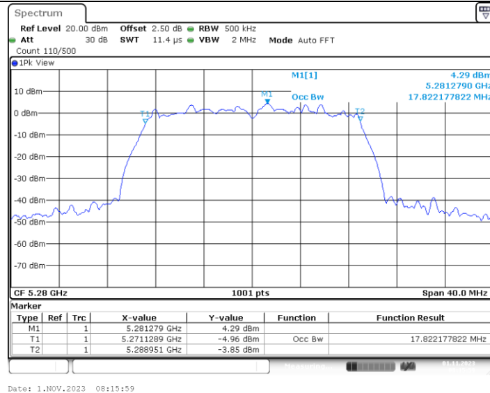
11N20MIMO_Ant2_5280
