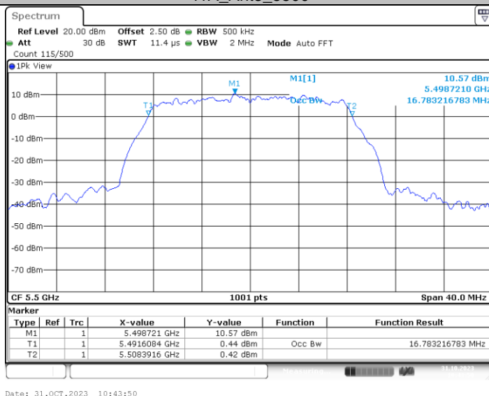
11A_Ant4_5500
