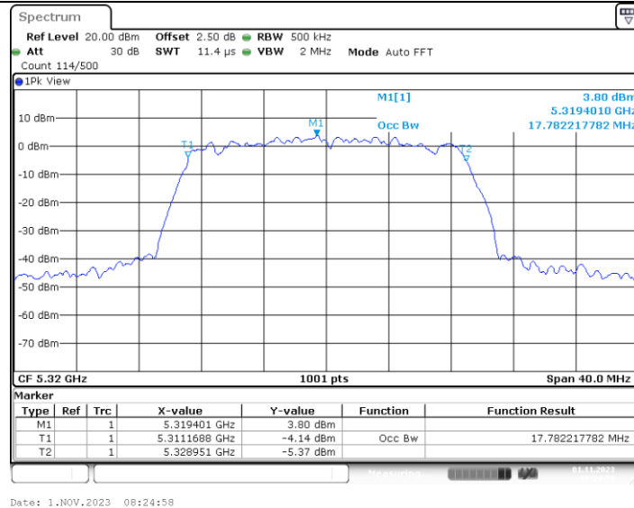
11N20MIMO_Ant4_5320
