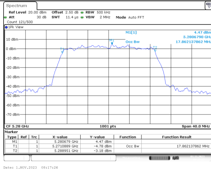
11N20MIMO_Ant3_5280
