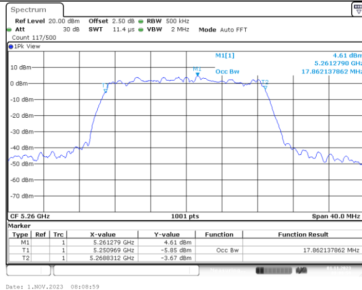
11N20MIMO_Ant3_5260
