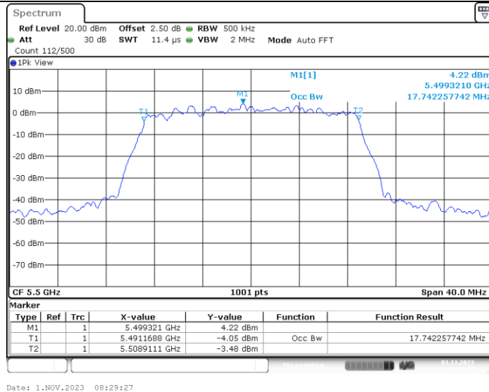
11N20MIMO_Ant3_5500
