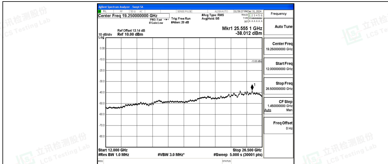
Band5-3MHz-QPSK-20525-1-0-Low-12000-26500--38.01-PASS
