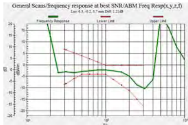
GSM850
