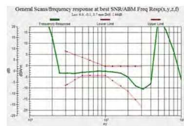
WCDMA1700/2100, Antenna 1
