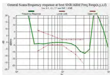
WCDMA850, Antenna 2
