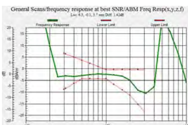
WCDMA1900, Antenna 1
