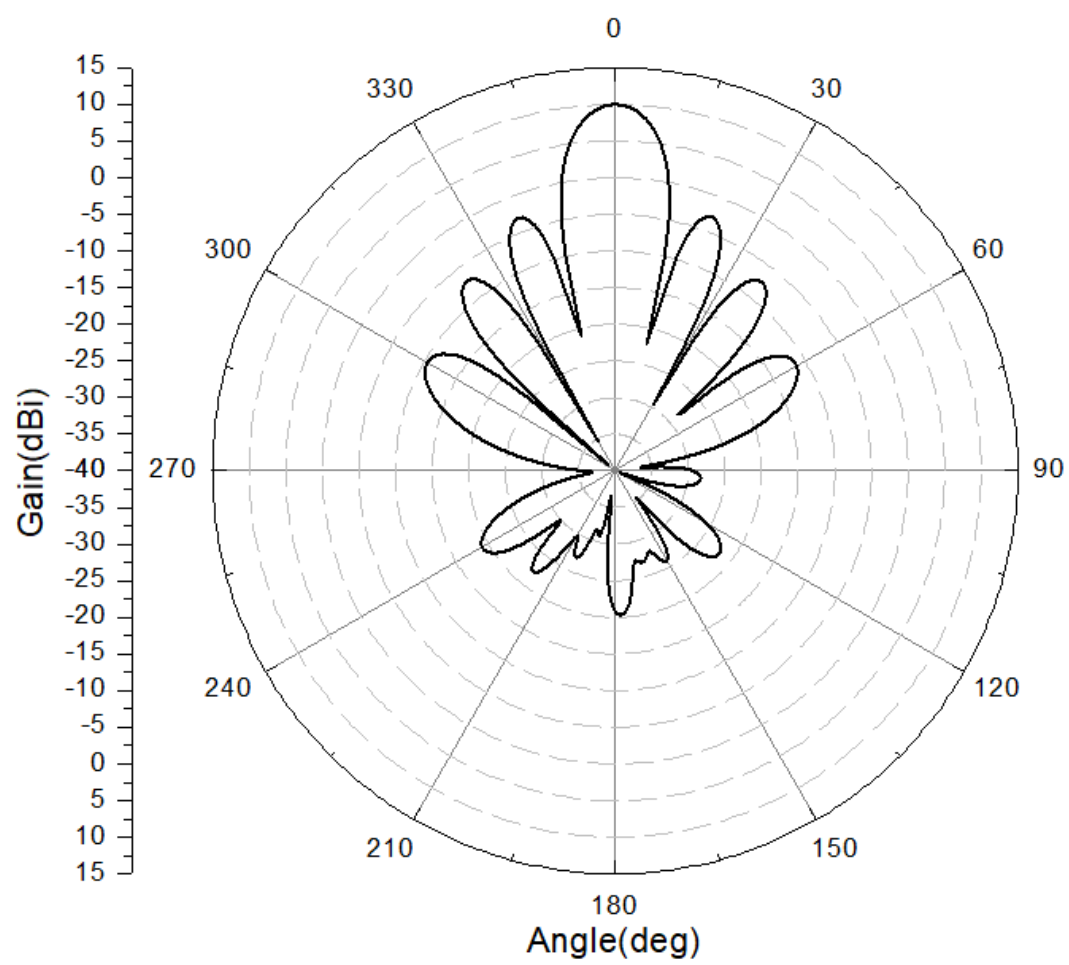
b) H 面
