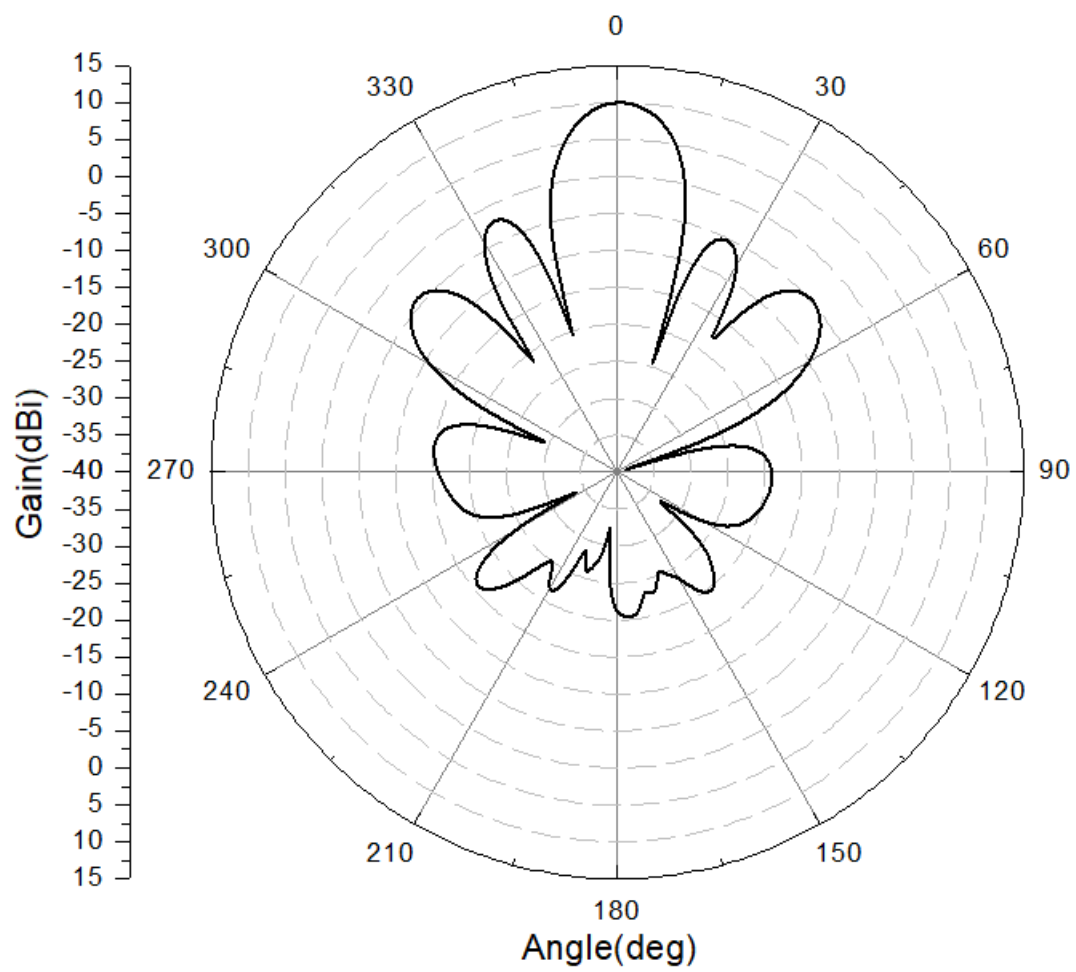
a) E 面
