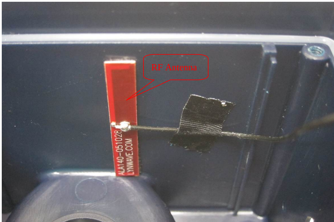
EUT 10 RF Antenna 1
