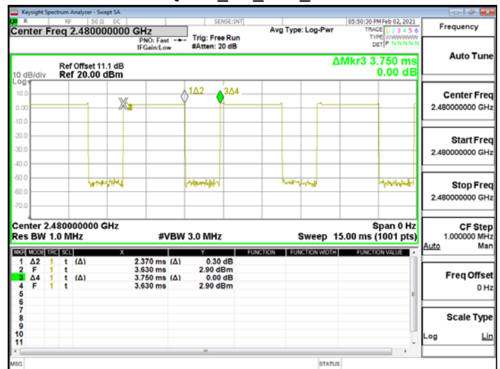
\pi /4DQPSK_2M_DH5_2480MHz
