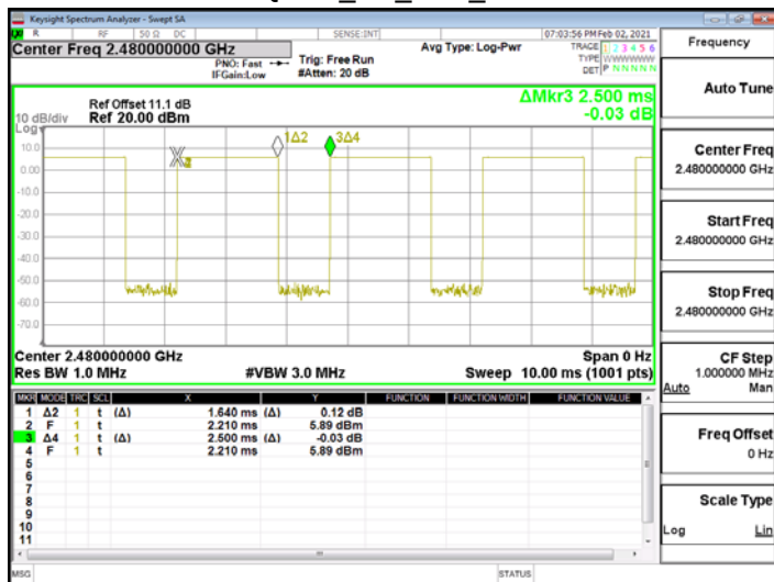
\pi /4DQPSK_2M_DH3_2480MHz
