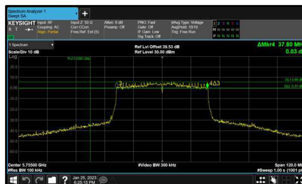
Figure 238 - 802.11ax HE40 SU Maximum 6 dB EBW
