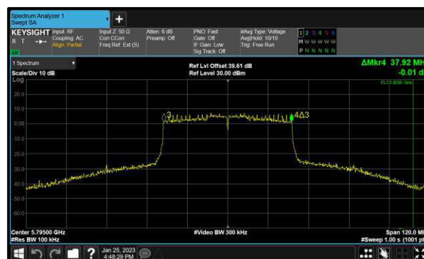
Figure 210 - 802.11ax HE40 SU Maximum 6 dB EBW
