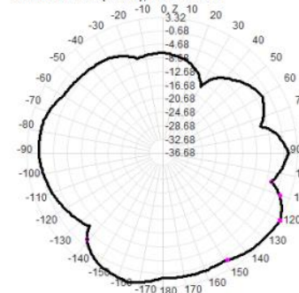
2500.0MHz Total(E2-YZ), Max= 3.32dBi
