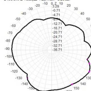
2480.0MHz Total(E2-YZ), Max= 3.29dBi
