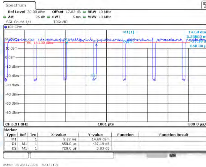
11AC40MIMO_Ant2_5310
