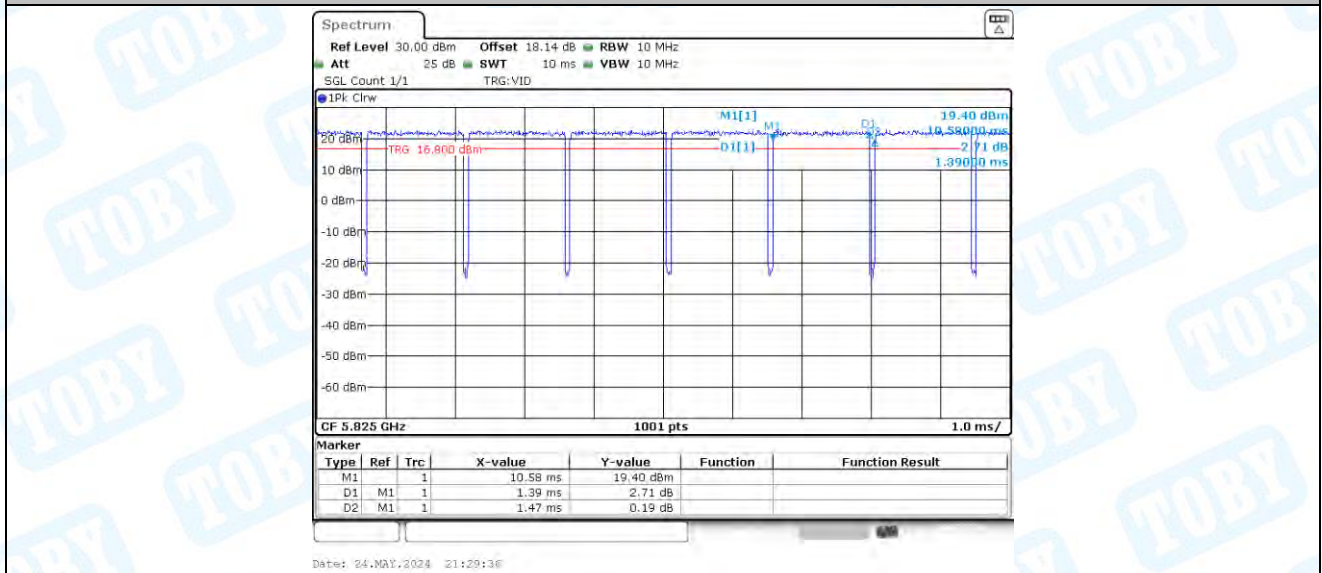
11A_Ant2_5825
