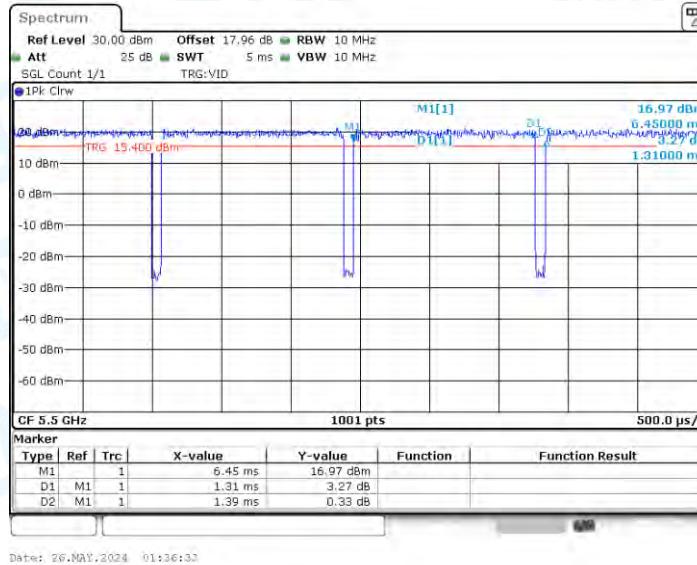
11AC20MIMO_Ant2_5500
