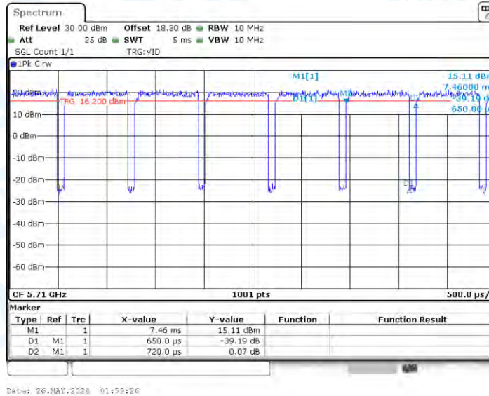
11AC40MIMO_Ant2_5710
