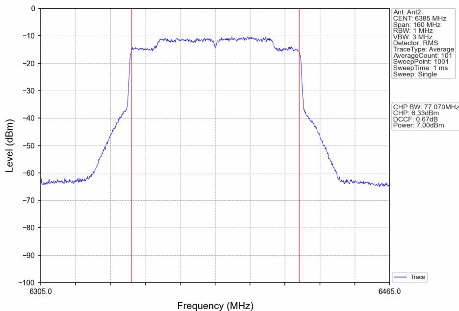
802.11ax(HEW80)_HCH_6385MHz_RU996_Left_Ant2_NTNV
